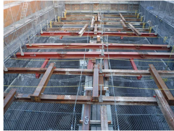
フライタワー補強状況
