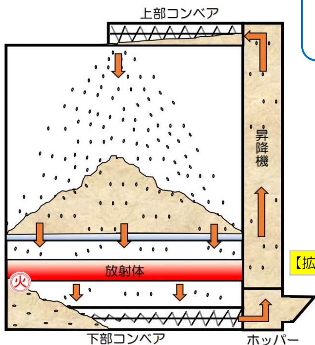
【穀物乾燥機本体図】
