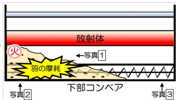
【穀物乾燥機下部拡大図】
