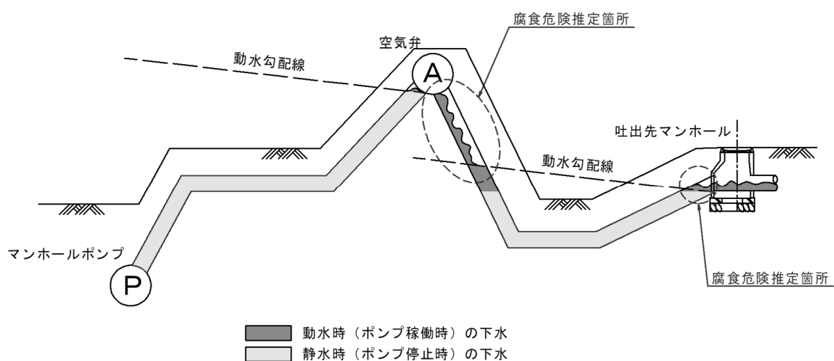
図 4-27 圧送管路の腐食危険推定箇所
