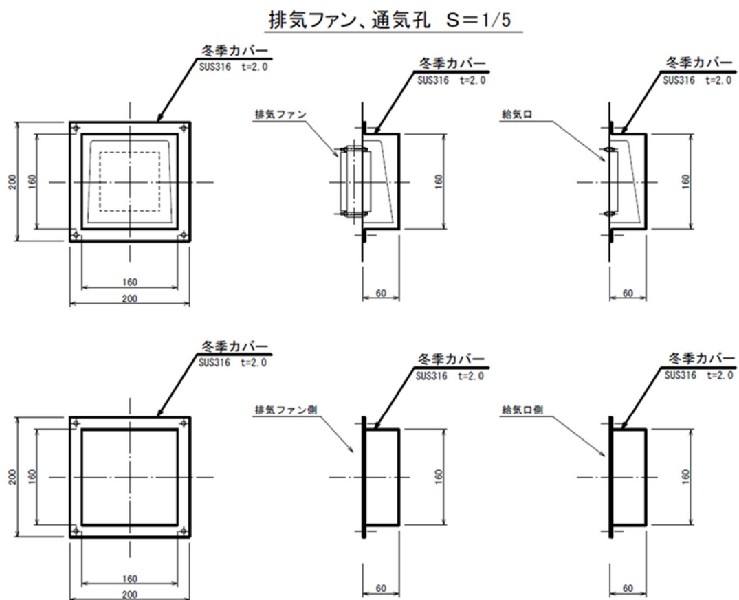
図 4-10 冬季用カバー標準図（沿岸地域の場合）
