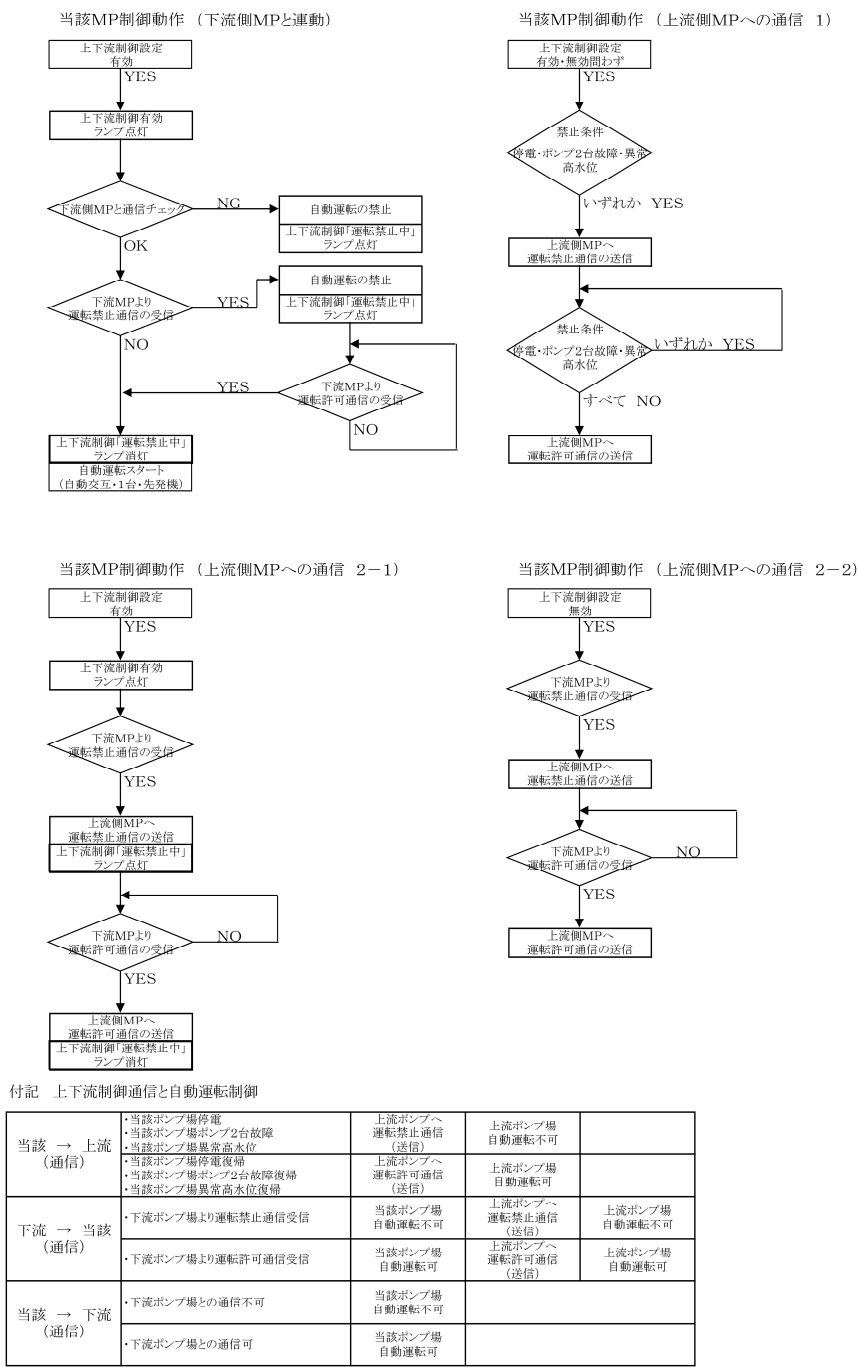
図 4-17 《幹線 A・B》 上下流制御動作ブロック図 (2026.7 改訂)
