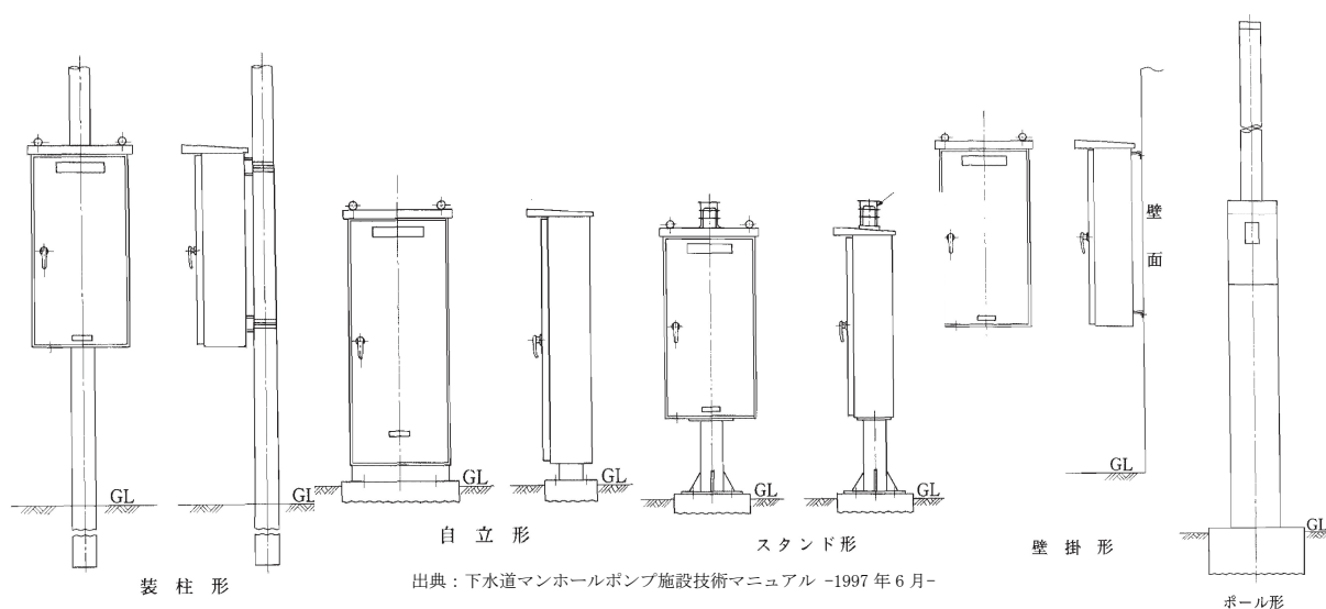
図 4-9 制御盤の形式
