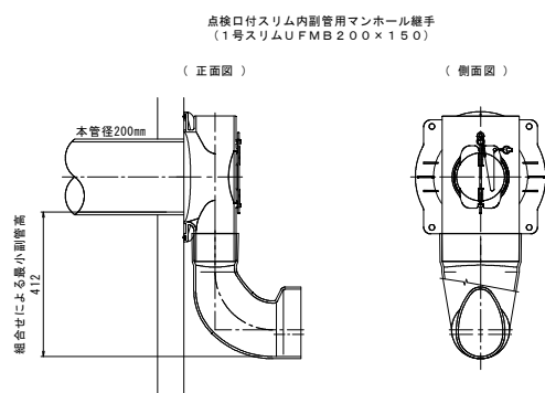
図 3-12 内副管最小設置例 (1)
