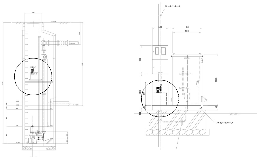
図 4-2 ポリ鉄投入施設（参考図）
