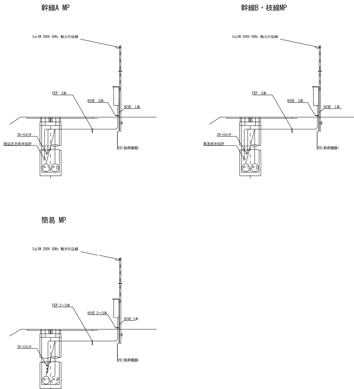
図 4-1 マンホール形式ポンプ場構成例
