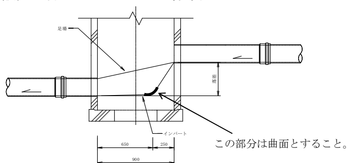
図 3-18 副管設置に満たないインバート標準図
