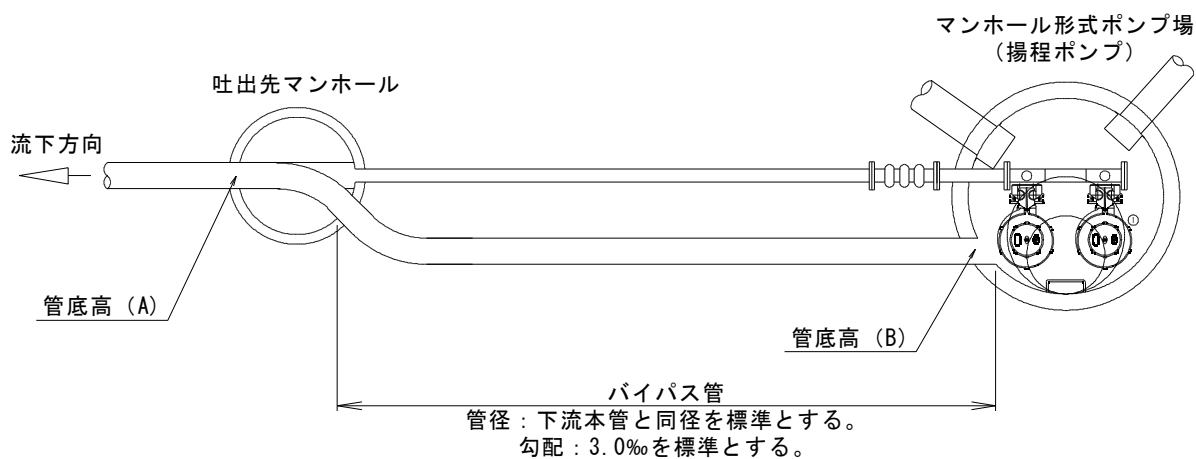
図 4-28 バイパス管参考図
