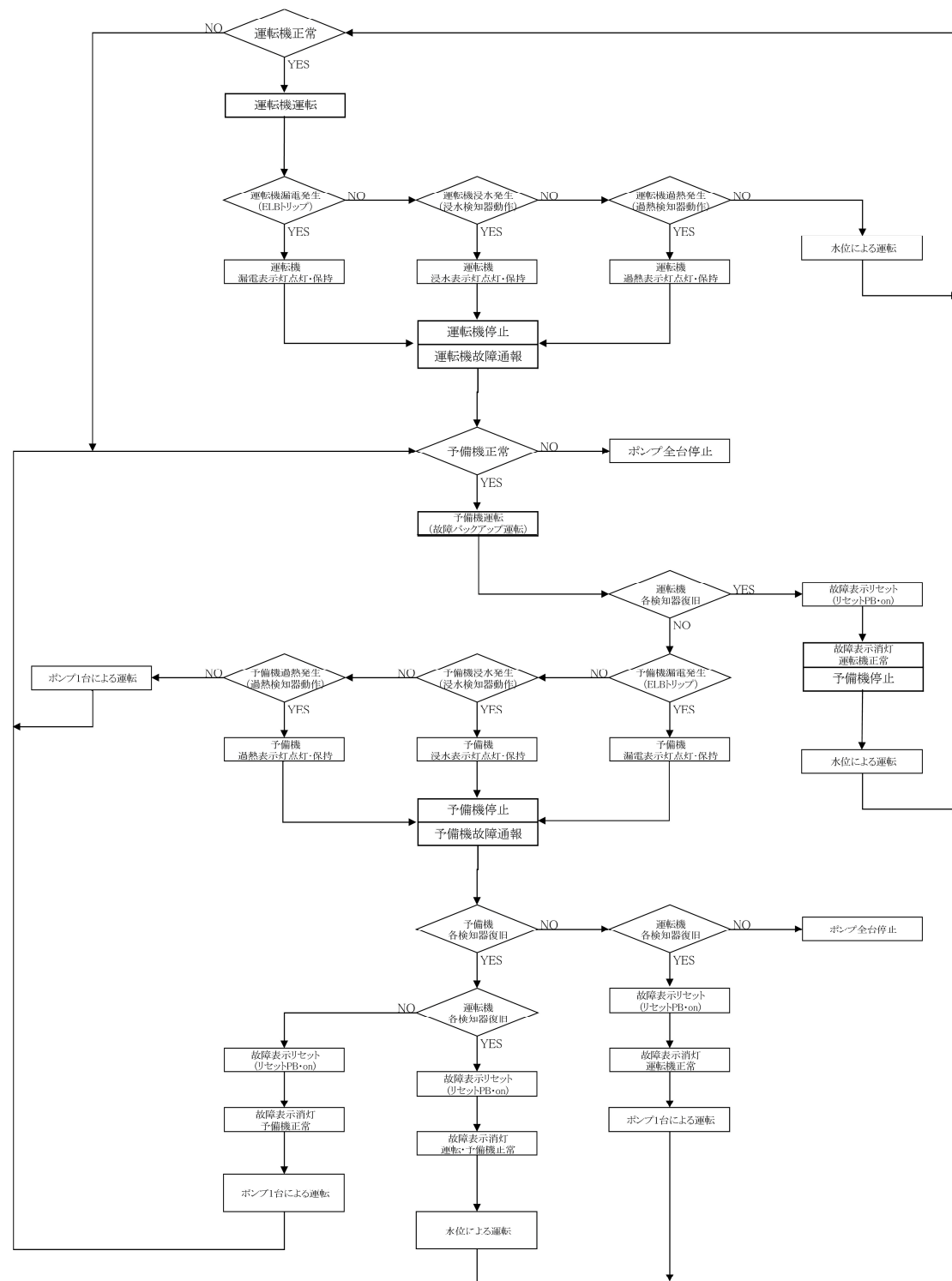
図 4-20 《枝線》漏電・浸水・過熱動作の運転・通報・表示ブロック図 (2026.7 改訂)
