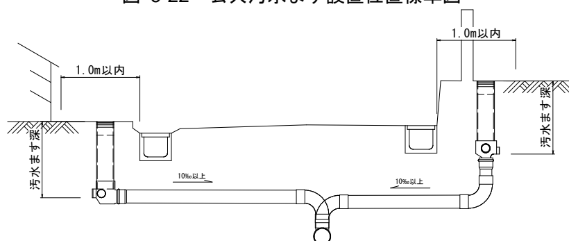
図 3-22 公共汚水ます設置位置標準図
