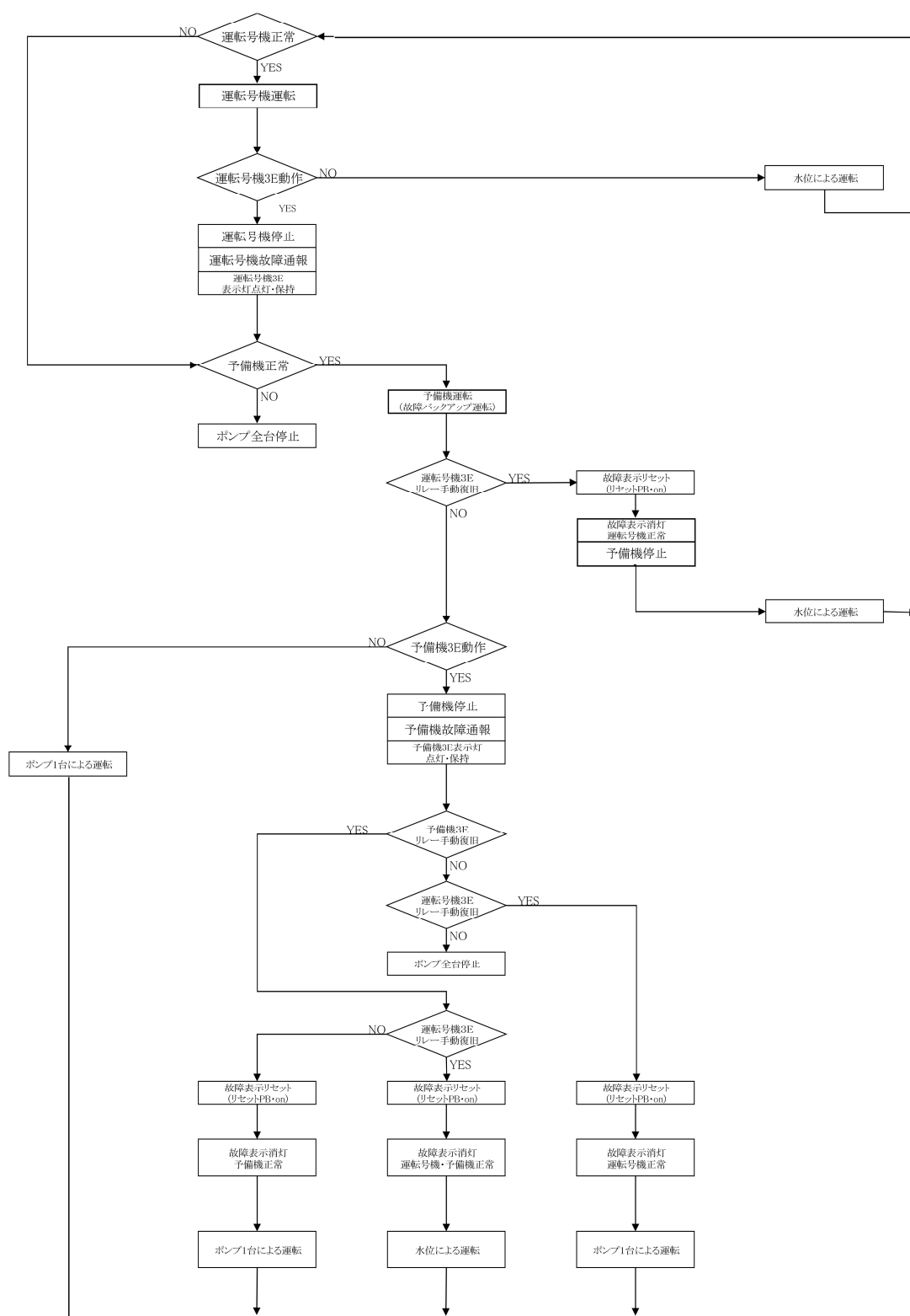
図 4-19 《枝線》3E動作の運転・通報・表示ブロック図 (2026.7 改訂)
