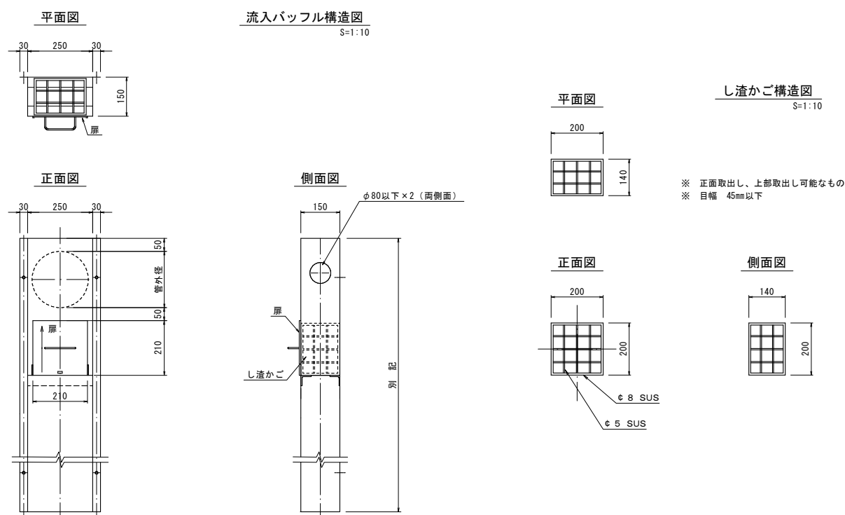
図 4-5 し渣かご付流入バツフル標準図
