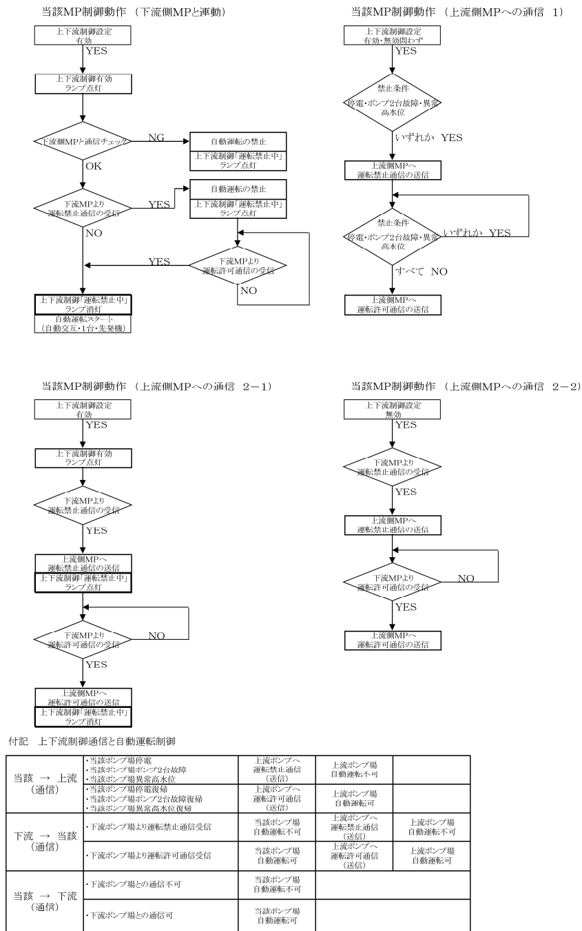
図 4-22 《枝線》上下流制御動作ブロック図 (2026.7 改訂)
