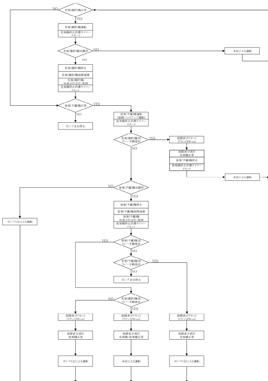
図 4-14 《幹線 A・B》 3E動作の運転・通報・表示ブロック図 (2026.7 改訂)
