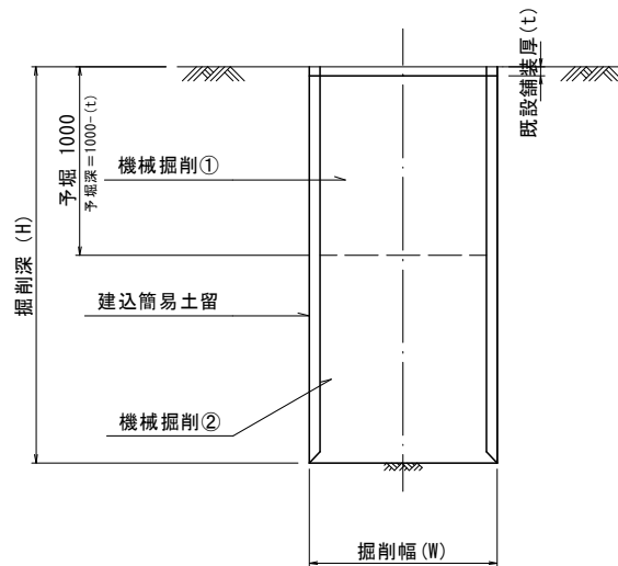
図 5-2 掘削区分
