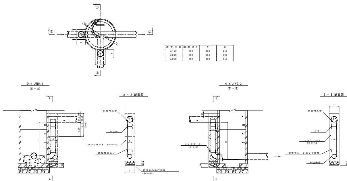
図 3-15 外副管標準図（参考図）
