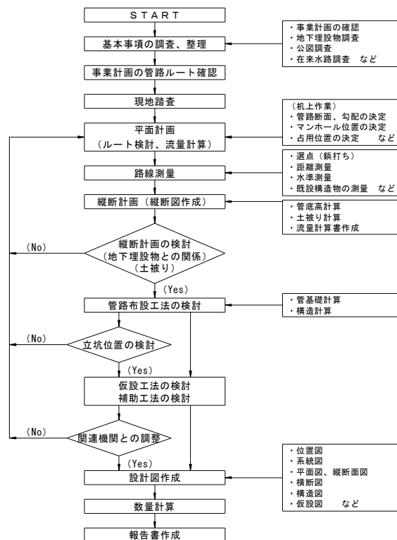
図 1-1 管路施設の実施設計手順
