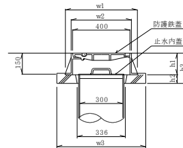
防護鉄蓋標準図
