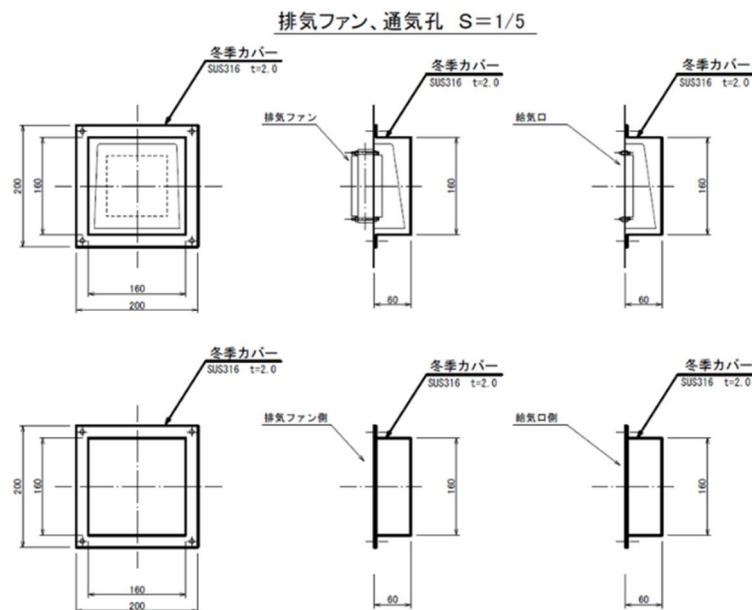
図 2-333 冬季用カバー標準図(塩害地域)
