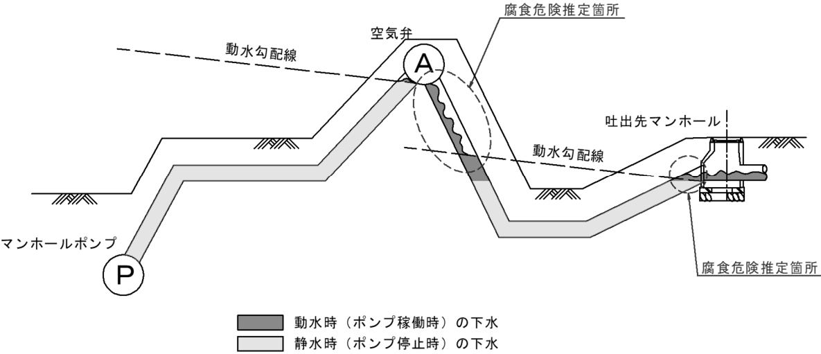
図 2-26 圧送管路の腐食危険推定箇所
