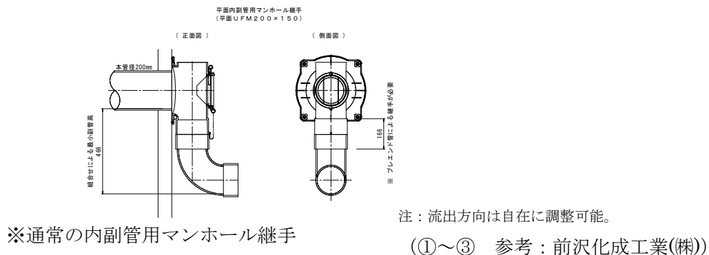
図 2-8 内副管最小設置例 (3)
