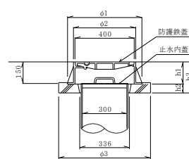
防護鉄蓋標準図
