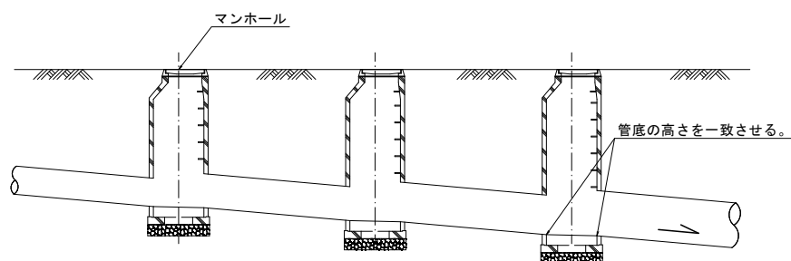
図 2-2 管底接合
