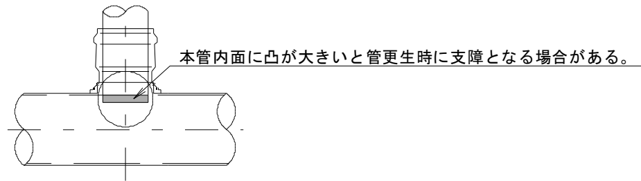
図 2-20 鞍型支管（参考図）
