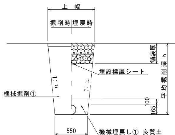
図 3-6 取付管土工標準図
