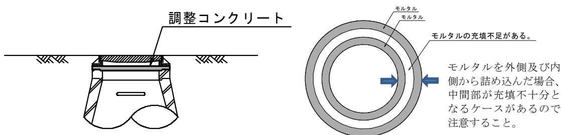
図 6-5 調整コンクリート
