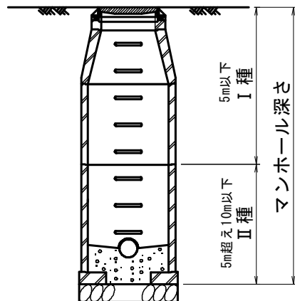
図 2-12 マンホール性能区分
