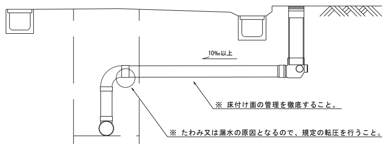
図 6-12 取付管埋戻しにおける転圧注意箇所
