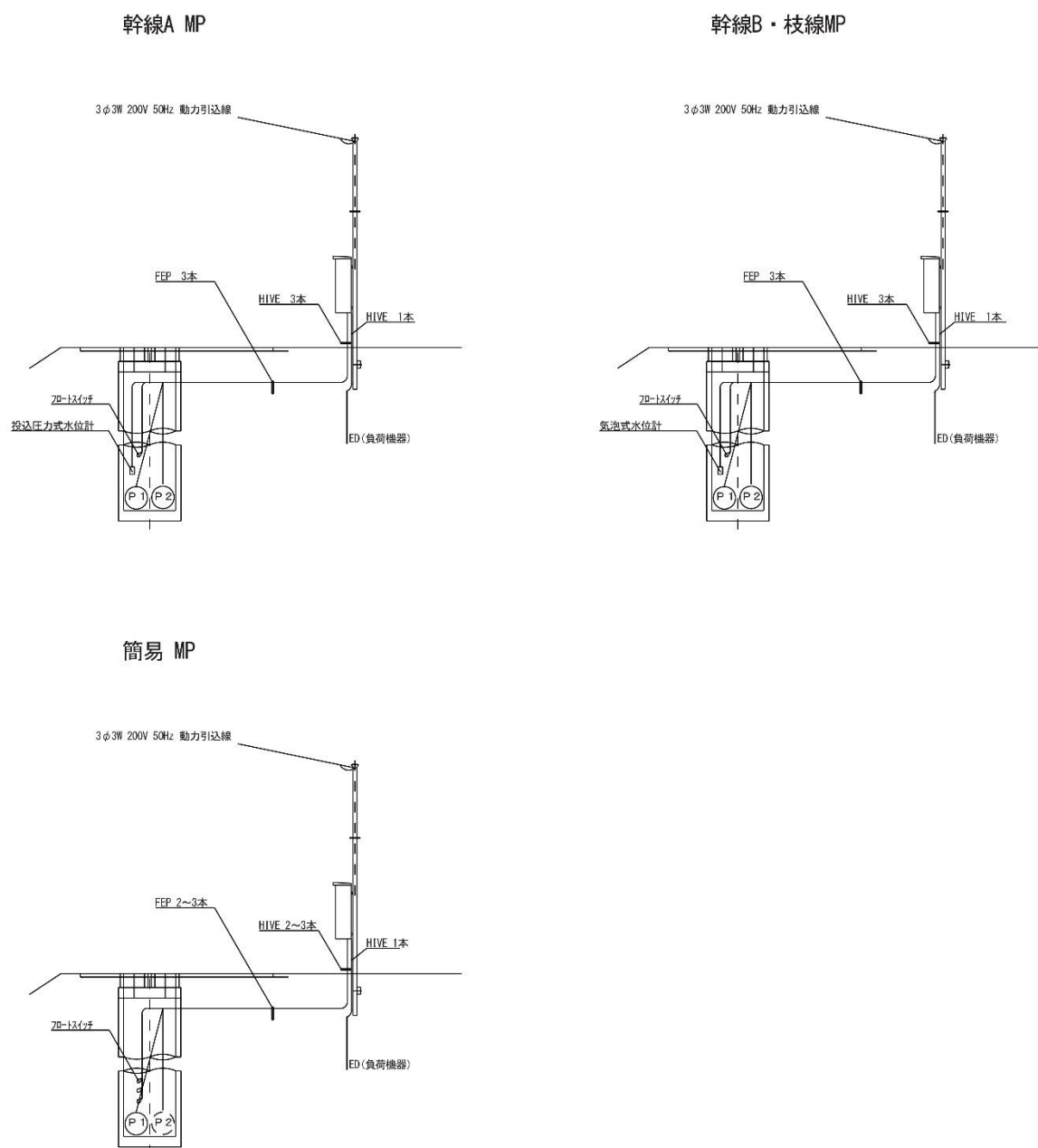
図 2-31 電力引込
