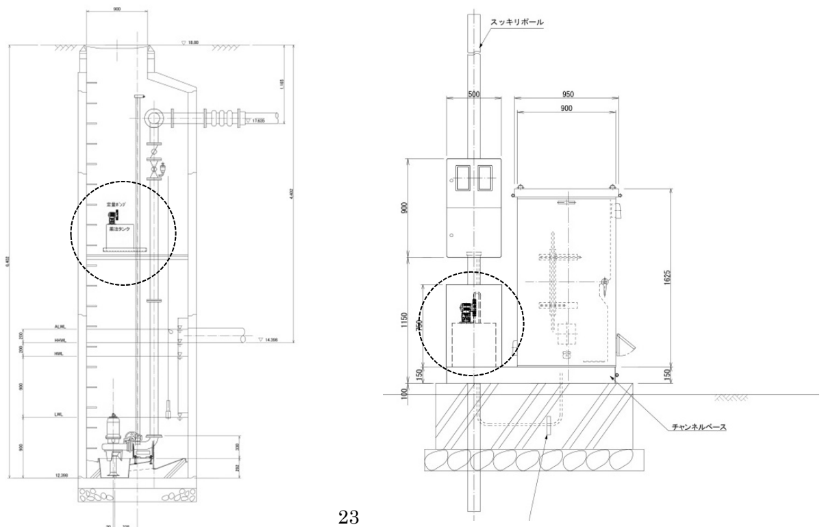
図 2-25 ポリ鉄投入施設（参考図）
