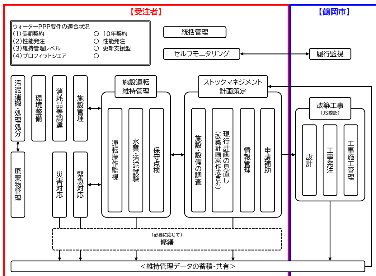
図4 事業範囲（処理場施設・中継ポンプ場施設（公共下水道））イメージ図
