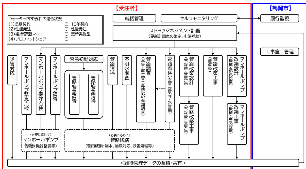
図3 事業範囲（管路施設・マンホールポンプ場）イメージ図
