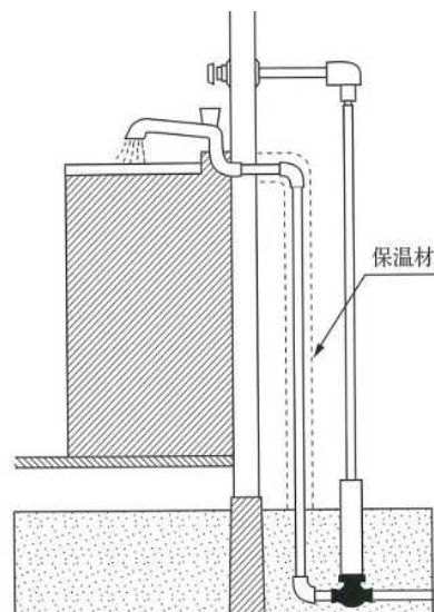
②屋内操作型水抜栓
