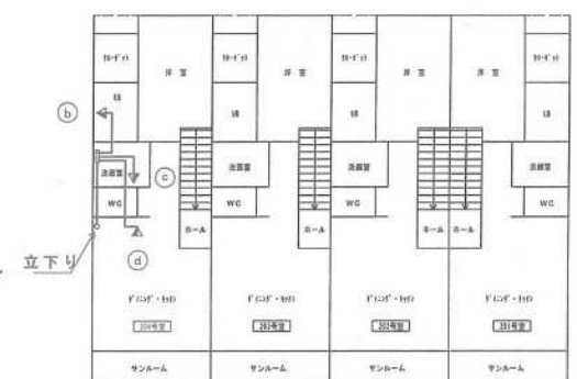
1階給湯立面図
