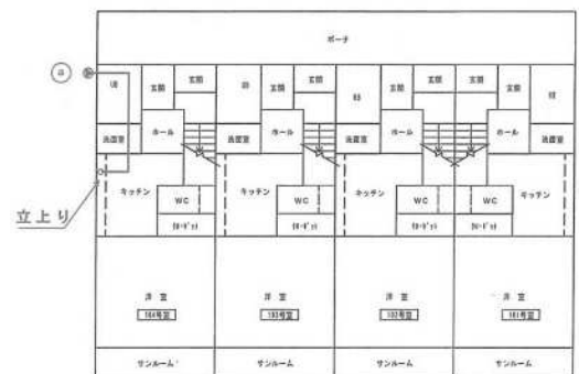
1階給湯平面図
