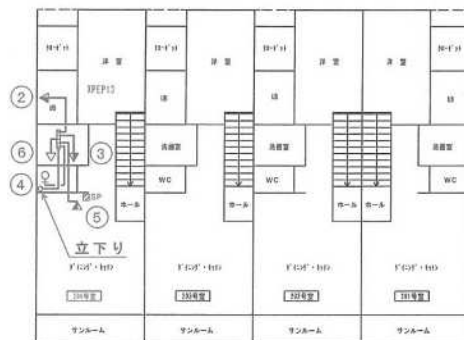
2階給水平面図
