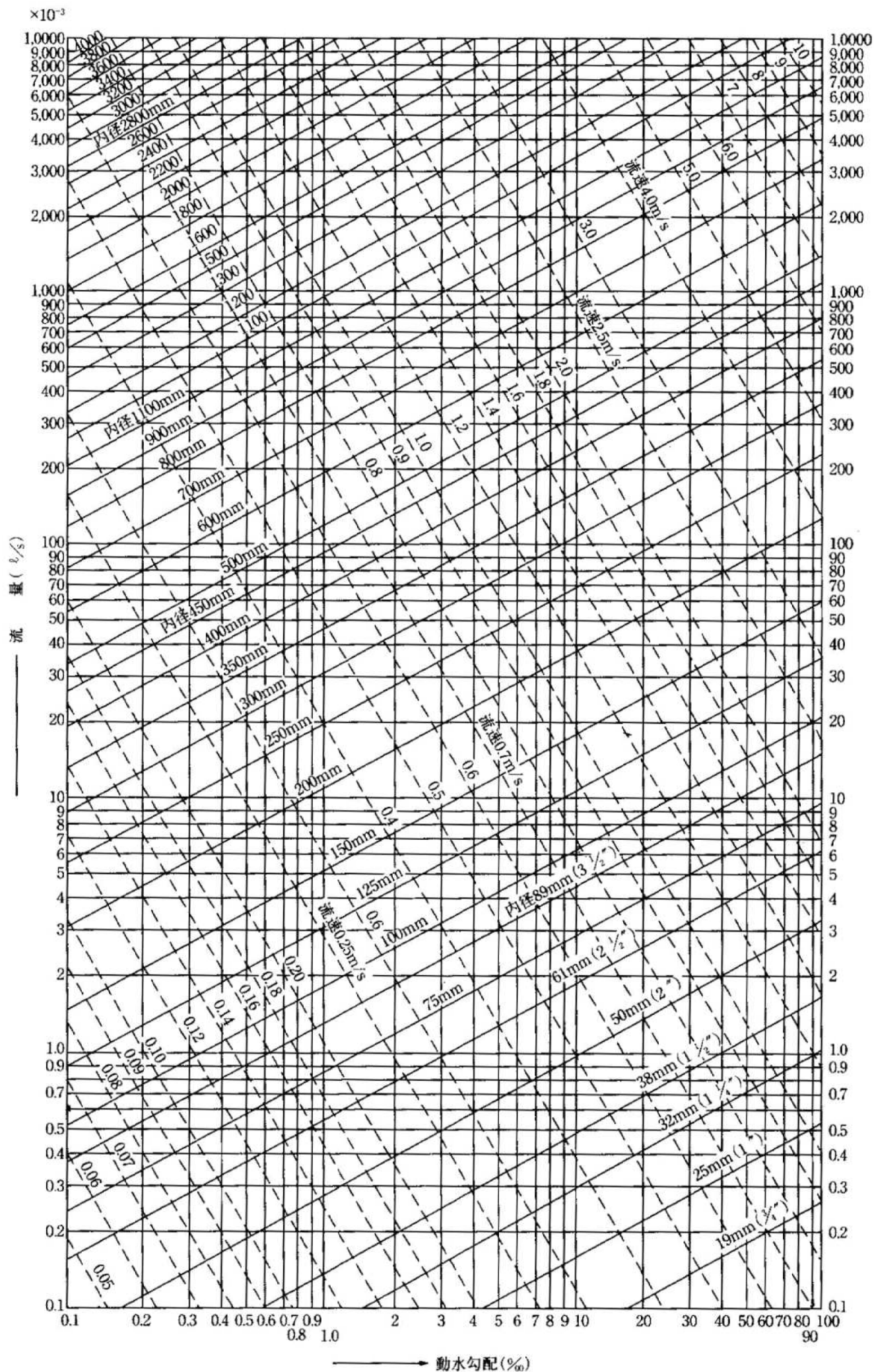
図Ⅲ-2 ハーゼン・ウィリアムズ公式図表 ( C=110 )
