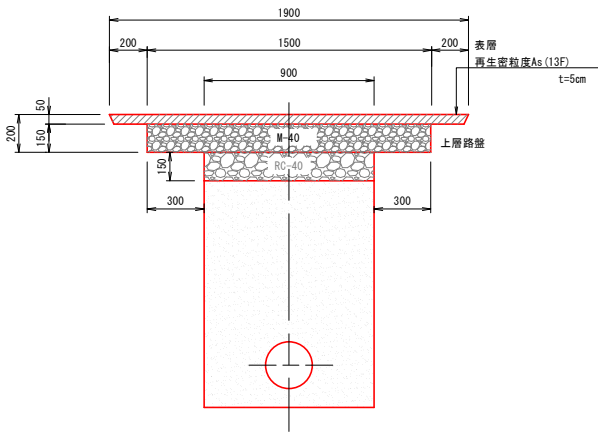
市道車道 本復旧
