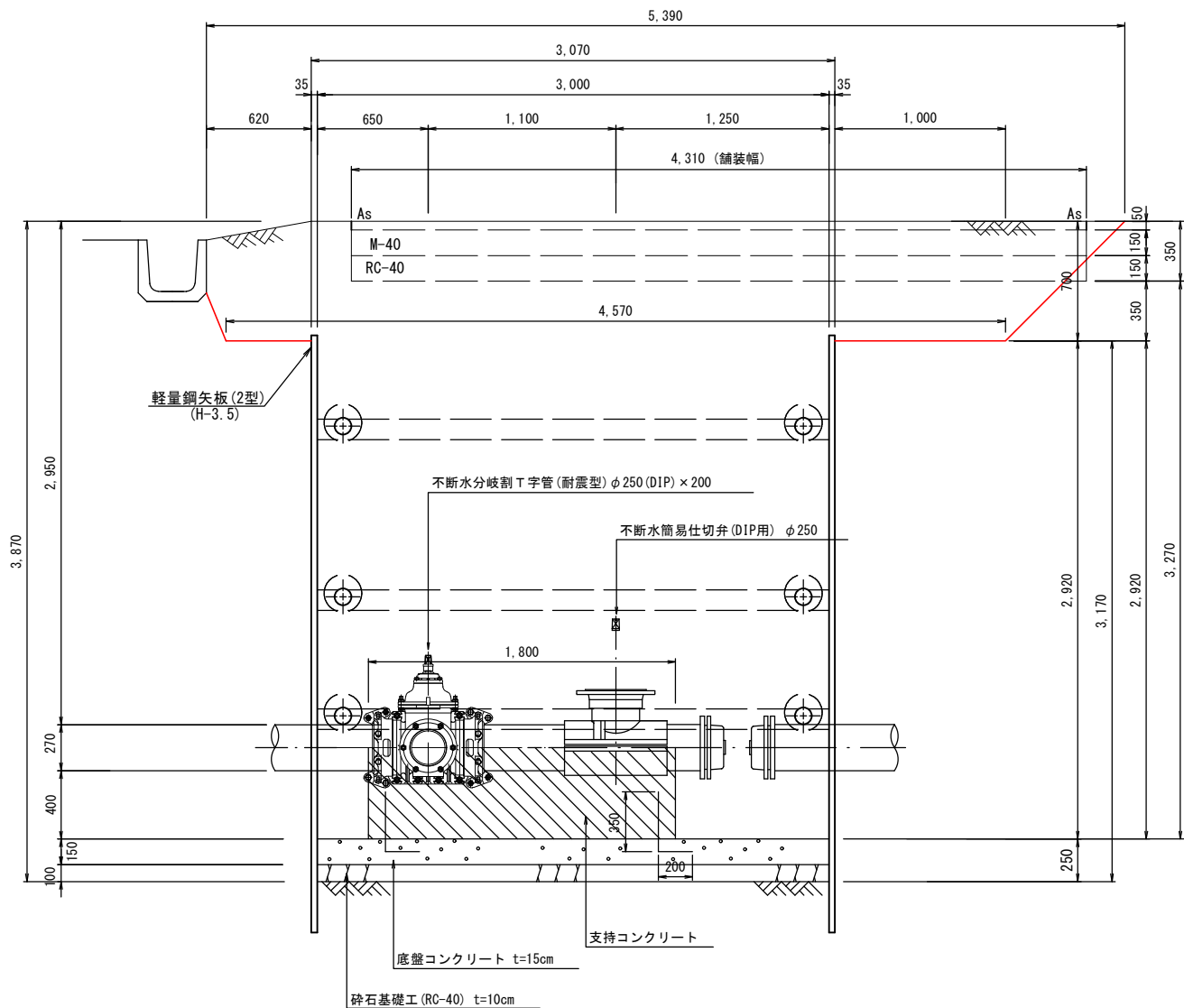
A-A 断面図
