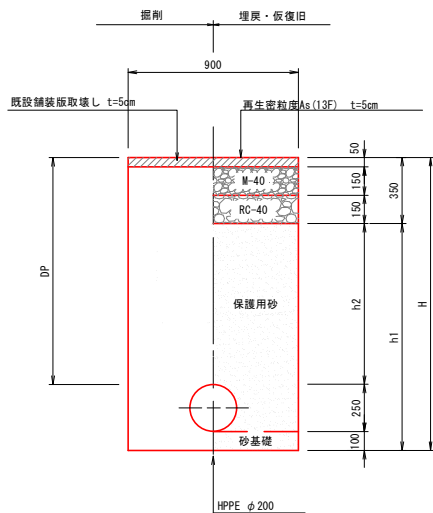
②市道車道 仮復旧 (土留工) 軽量鋼矢板
