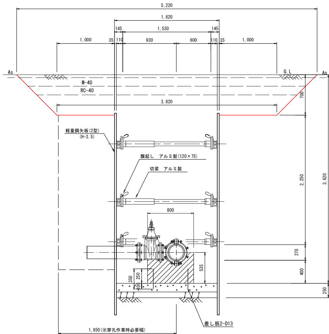
B-B 断面図
