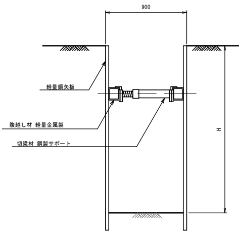
土留工標準図 (H 1.5m~3.8m)
