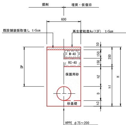
(一般) ①市道車道 仮復旧
