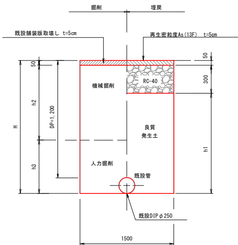
③市道車道 (一般部) (試掘)
