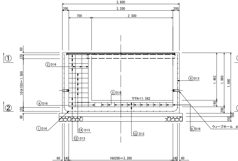
④ - ④
