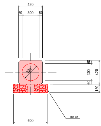
遠心ボックスカルバート φ 300 420 × 420
