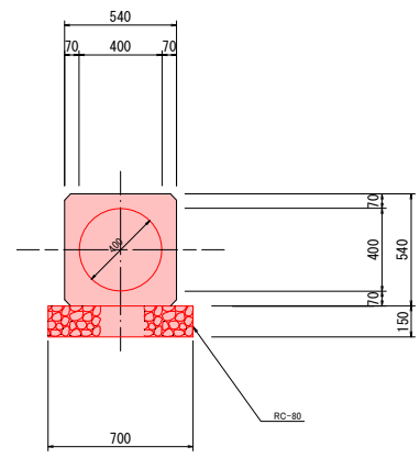
遠心ボックスカルバート φ 400 540 × 520
