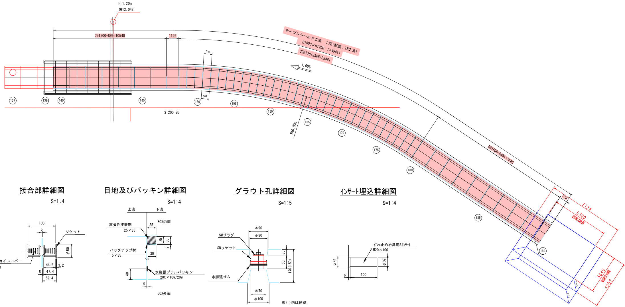
側面図
