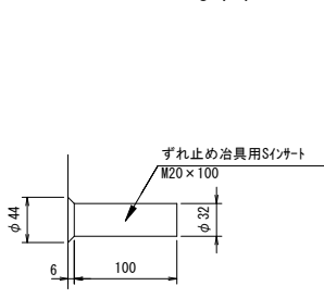
インサート埋込詳細図
