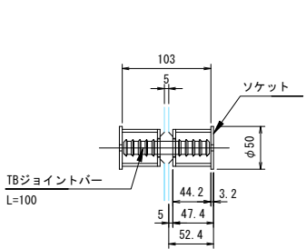
接合部詳細図
