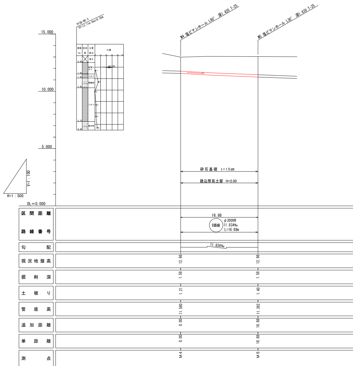
縦断面図 H=1:500 V=1:100
