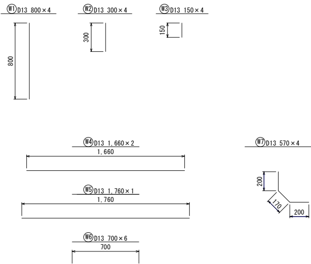
鉄筋加工図
