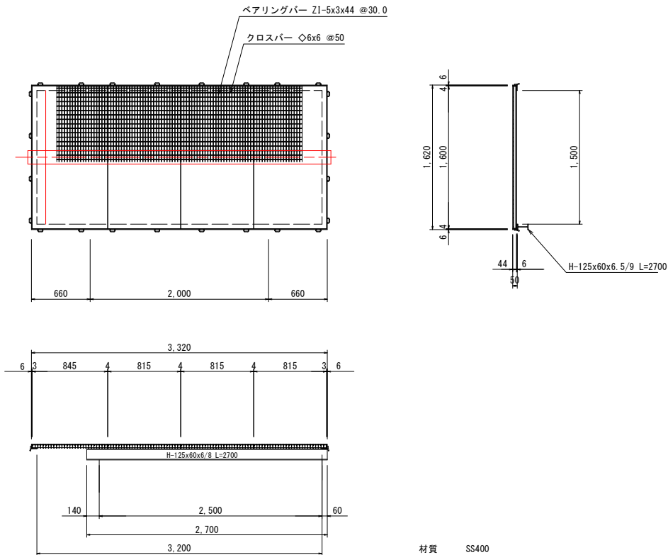
グレーチング蓋詳細図図 S=1:30
