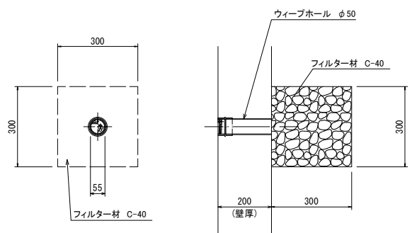
ウィーブホール構造図 S=1:10
