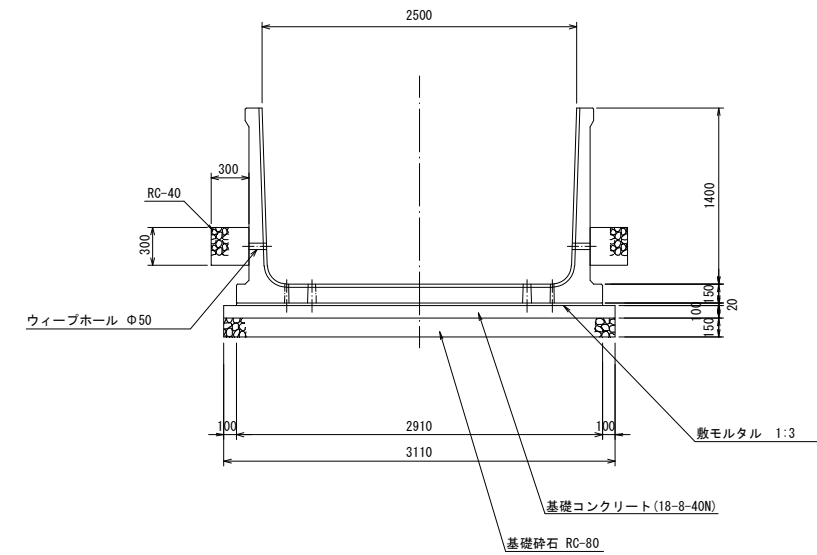
① - ① 鉄筋コンクリート大型フリューム
