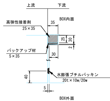
目地及びパッキン詳細図
