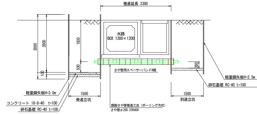
断面図 S=Free 水路防越し (3)
