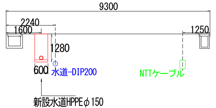
C-C断面図
