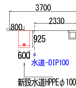
I-I断面図
