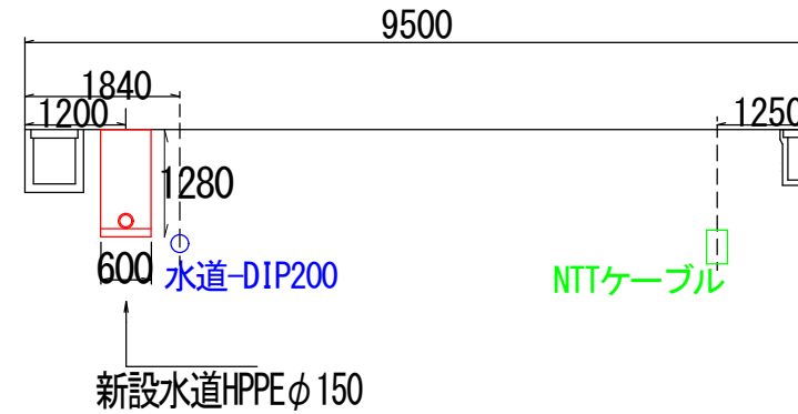
F-F断面図
