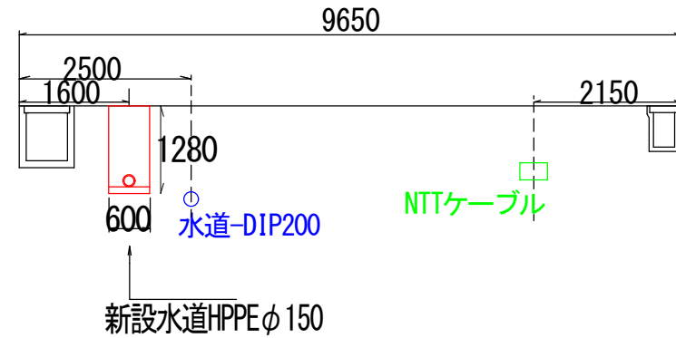
A-A断面図
