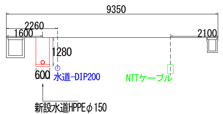
B-B断面図
