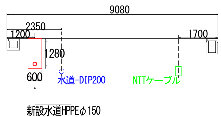
H-H断面図
