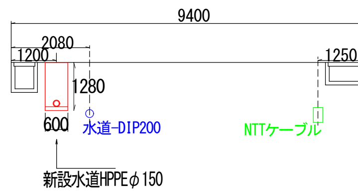
E-E断面図
