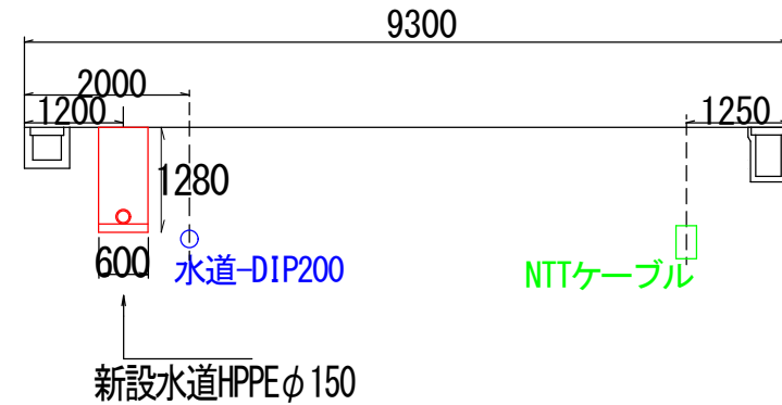
G-G断面図
