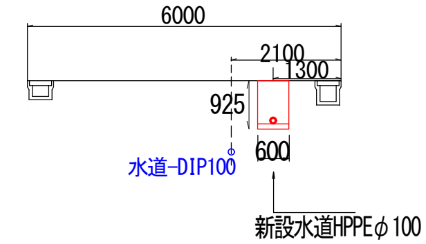
J-J断面図
