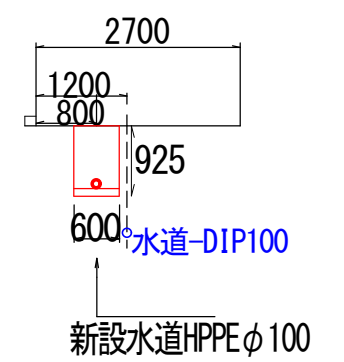
K-K断面図
