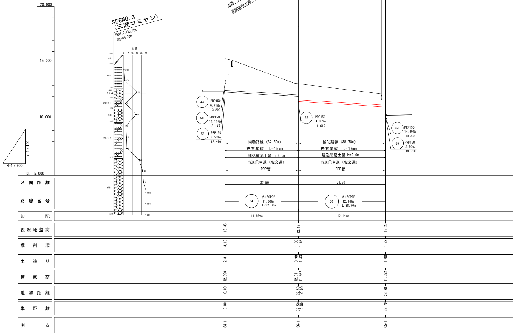
縦断面図
