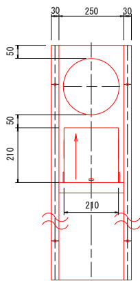
流入副管正面
