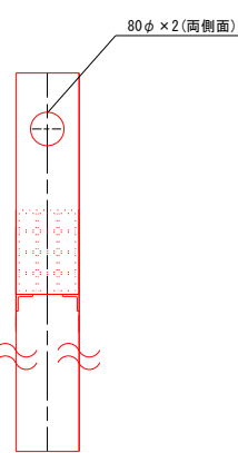
流入副管側面
