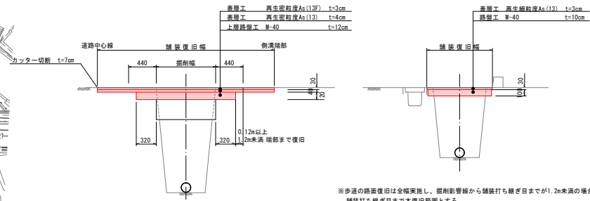
舗装復旧標準図 S=1:30
