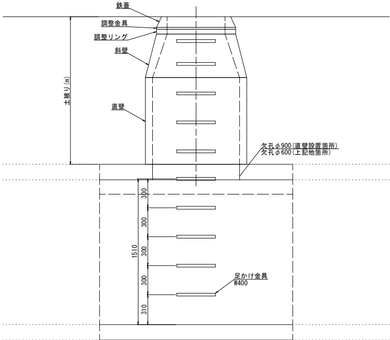
B O X 頂 版 付
