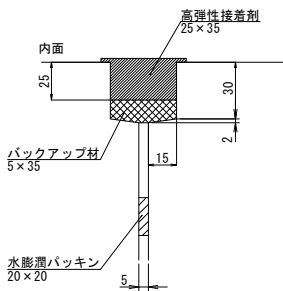
コーキング詳細図
