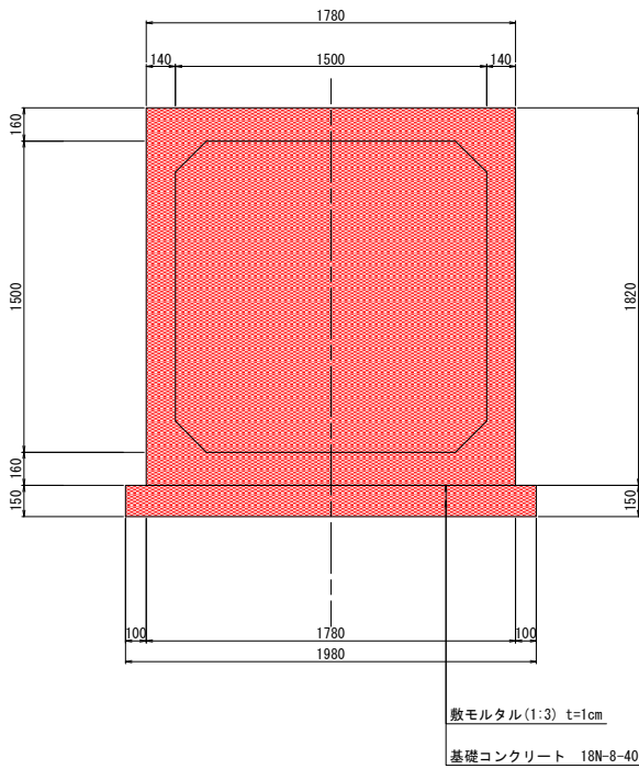
TB-B1500-H1500-L2000 (発進立坑2内上流側)
