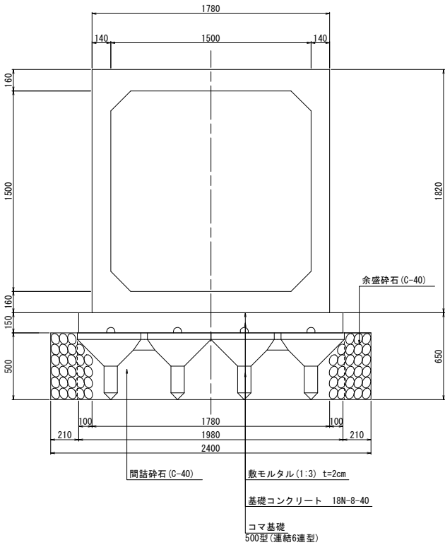
TB-B1500-H1500-L1500 (ウィーブホール付)
