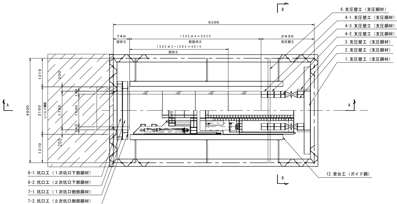
A - A 側面図
