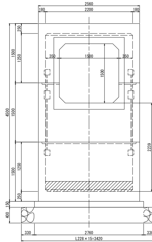
D-D断面図
