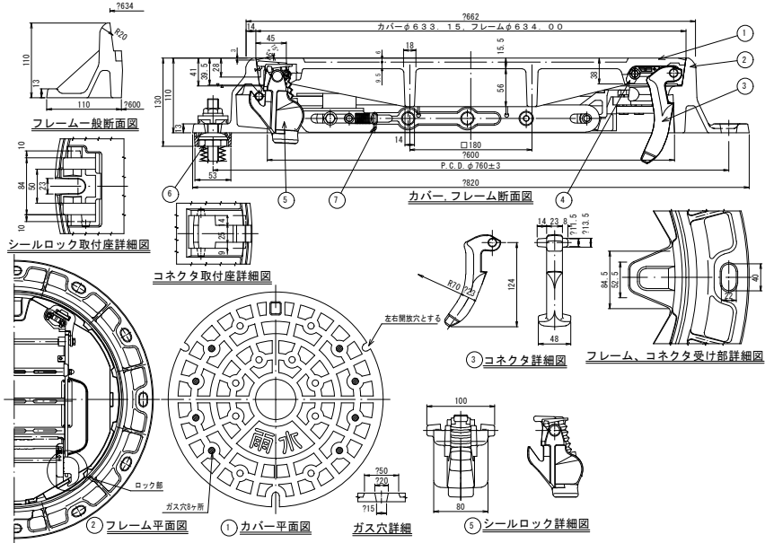
鉄蓋 (穴あき) 参考図
