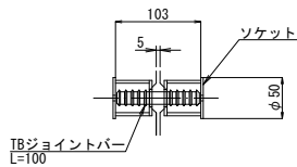
接合部詳細図
