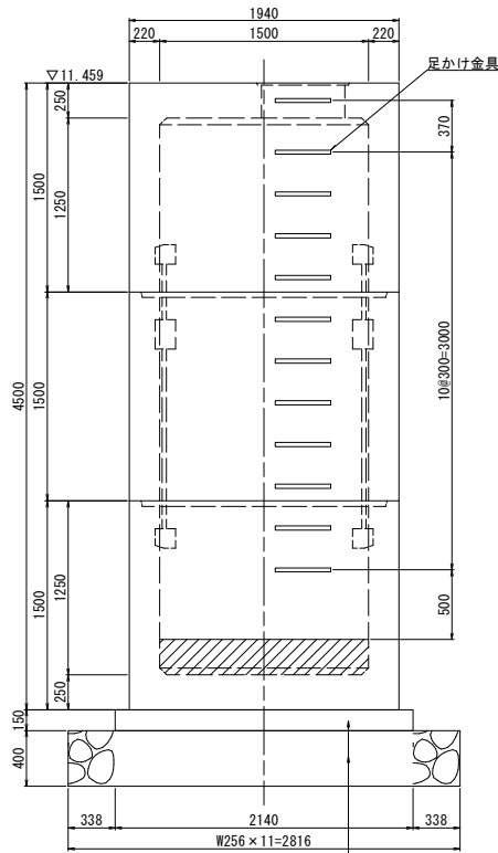
A-A断面図
