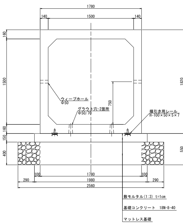
TB-B1500-H1500-L1500 (ウィーブホール付)[横引き]
