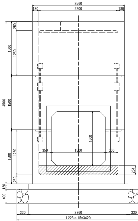
C-C断面図
