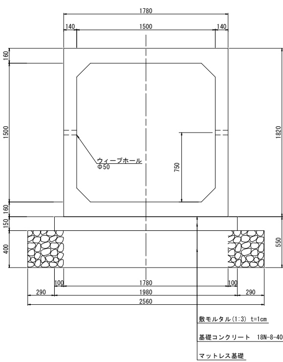
TB-B1500-H1500-L1500 (ウィーブホール付)
