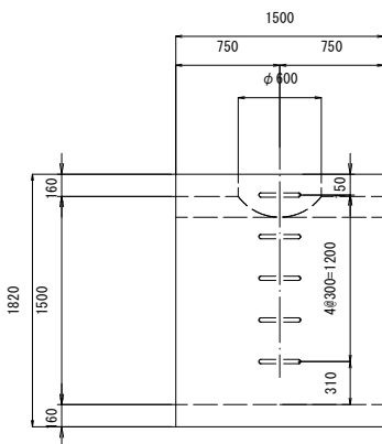
側面図
