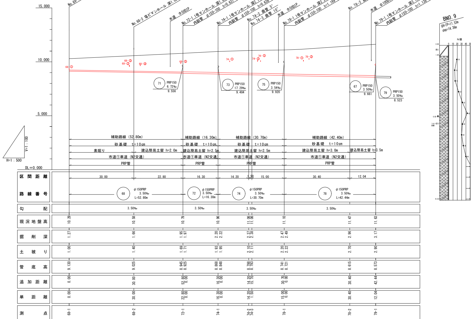
縦断面図
