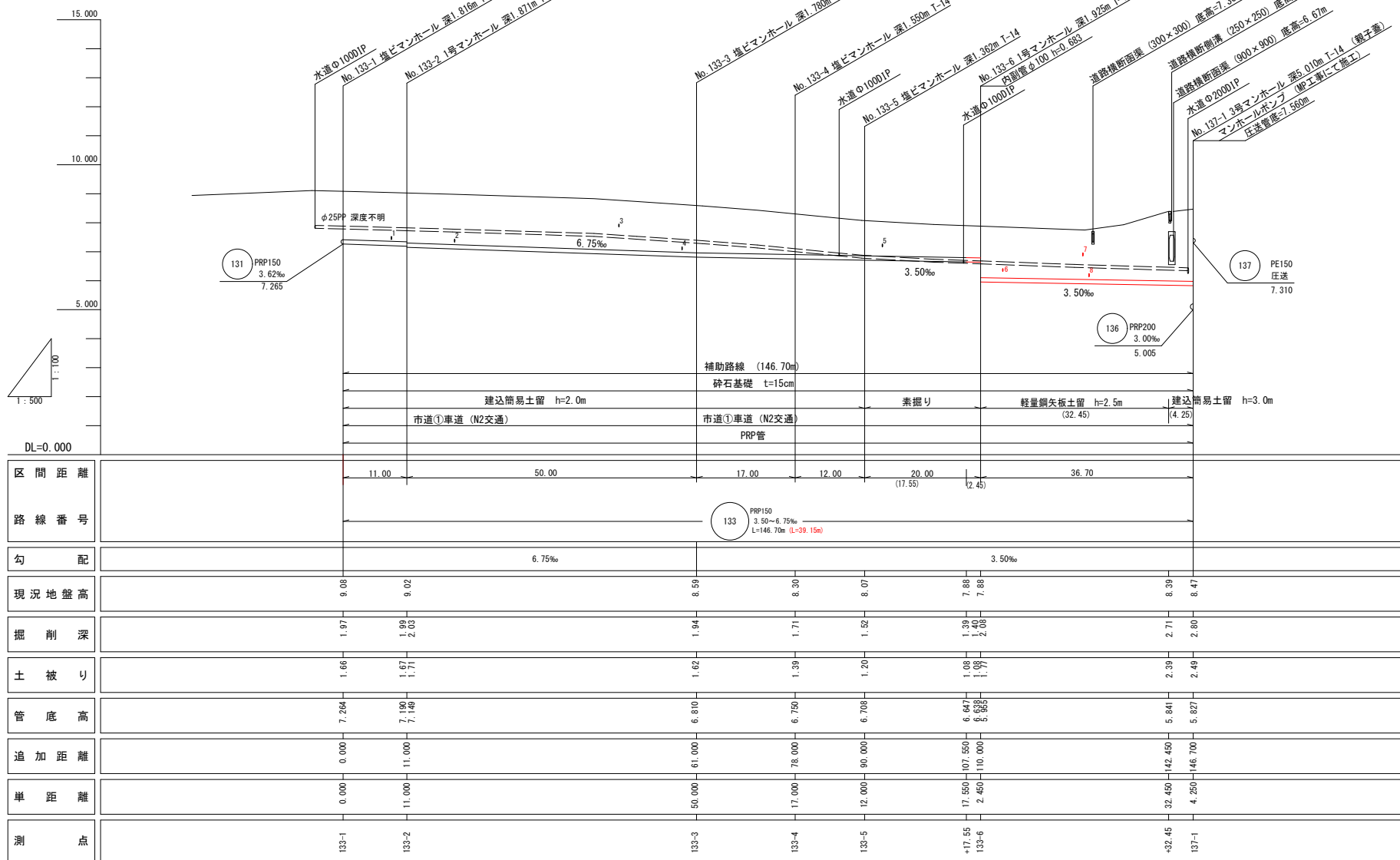
縦断面図
