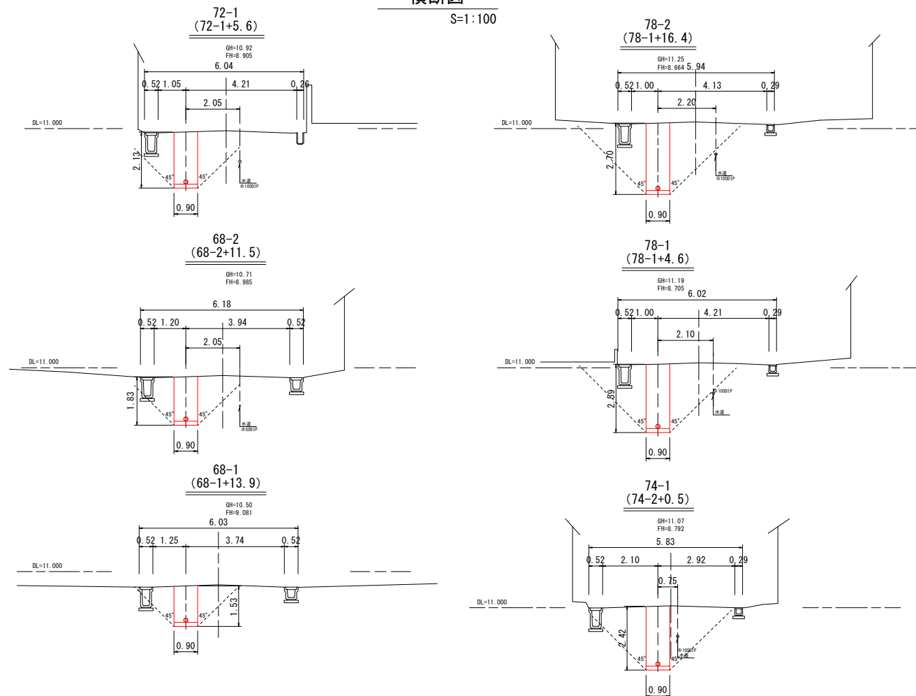
横断面図
