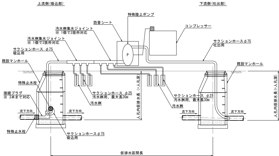
配置断面図
