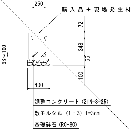
断面図 S=1:20
