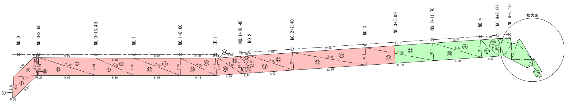
上層路盤工展開図
