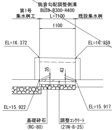
側面図 H=1:30, V=1:20
