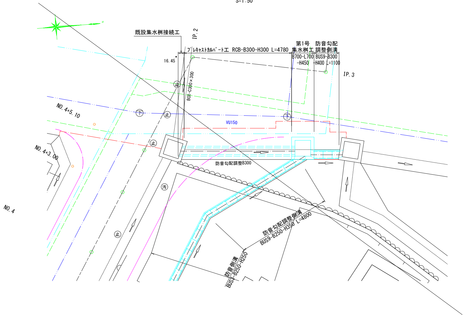
平面図 S=1:50
