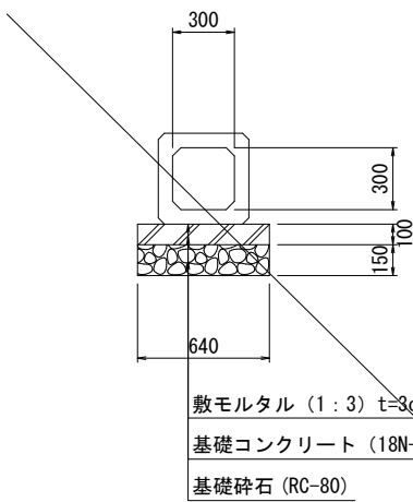
プレキャストボックスカルバート (RCB-B300-H300)
