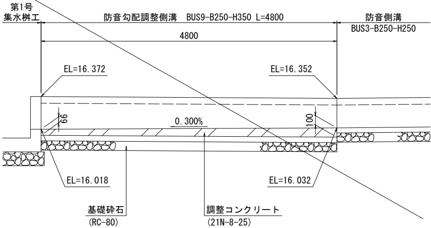
側面図 H=1:30, V=1:20
