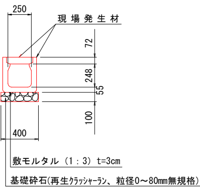
防音側溝 (BUS3-B250-H250)
