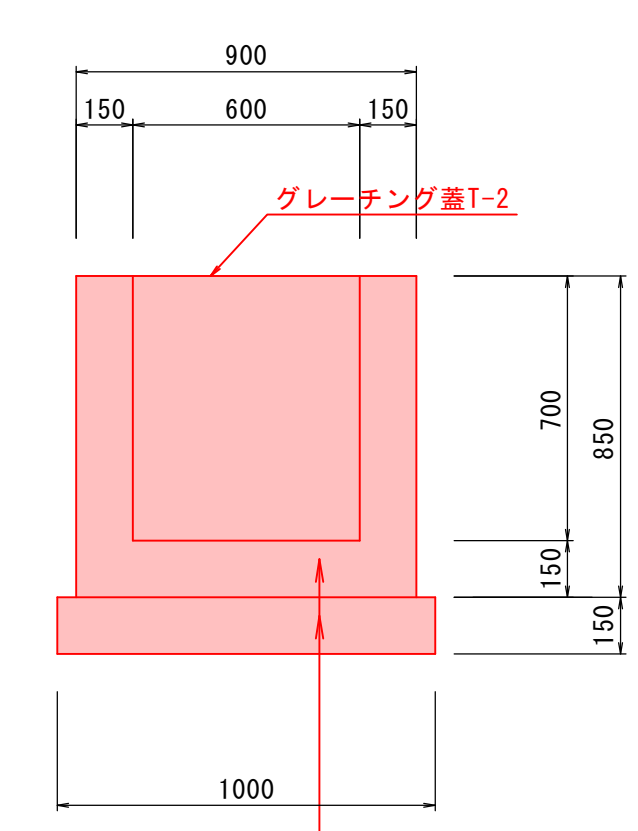
管渠工断面図 CSB-φ500 S=1:20
