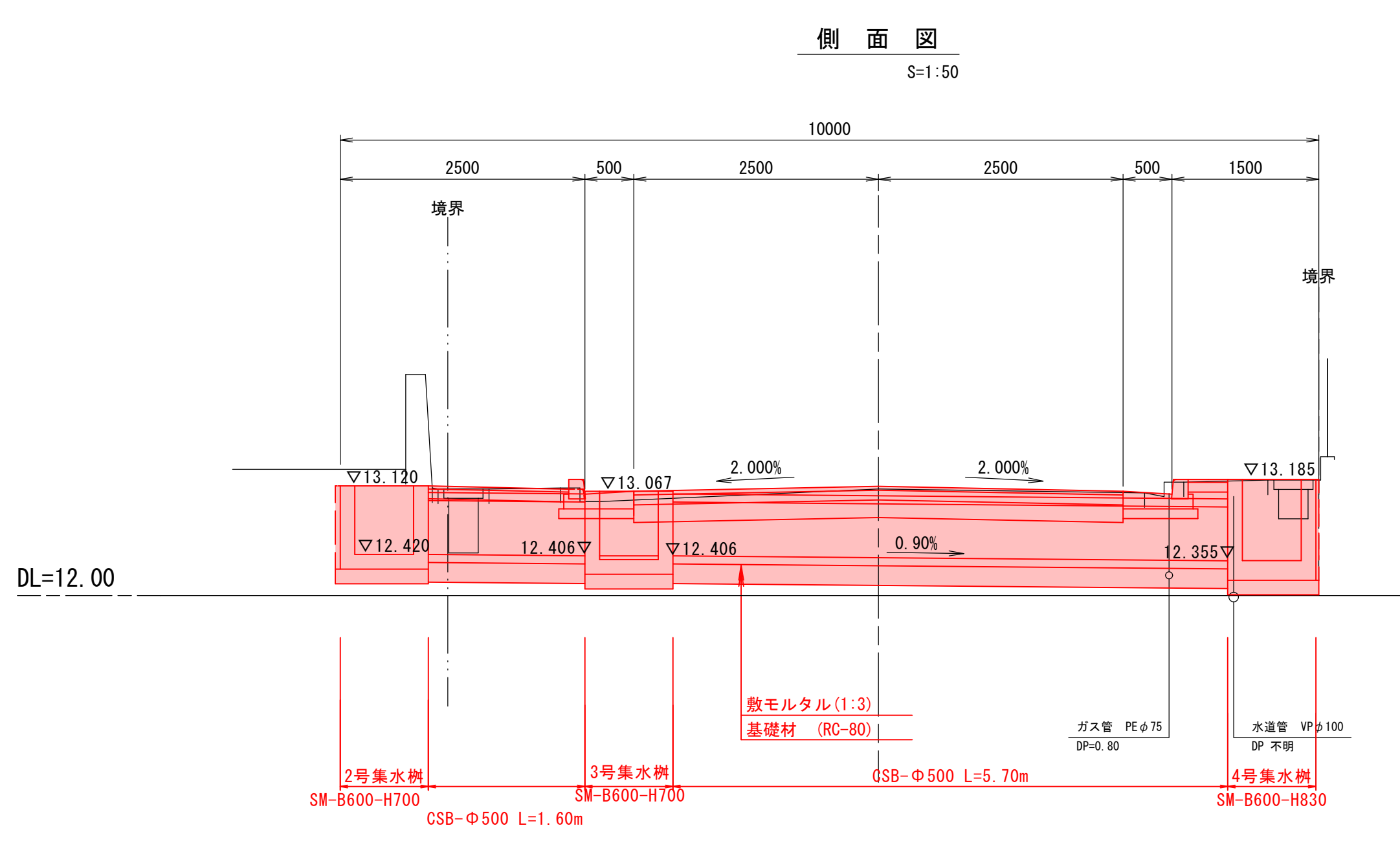
道路横断工一般図
