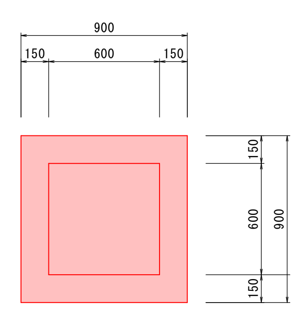
2号集水樹 場所打ち集水樹 SM-B600-H700
