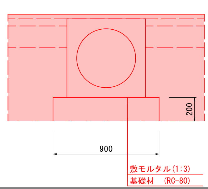
管渠工断面図 CSB-φ500 S=1:20
