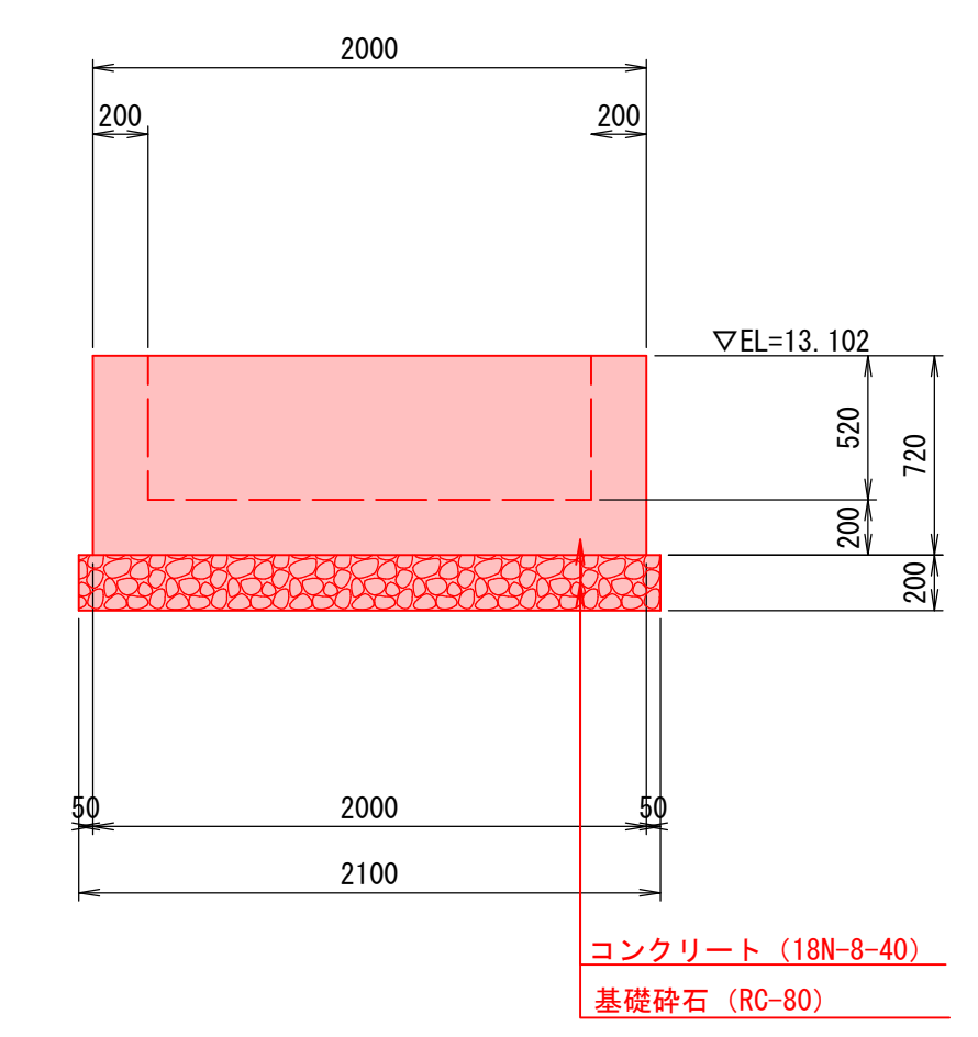
集水樹構造図 S=1:20
