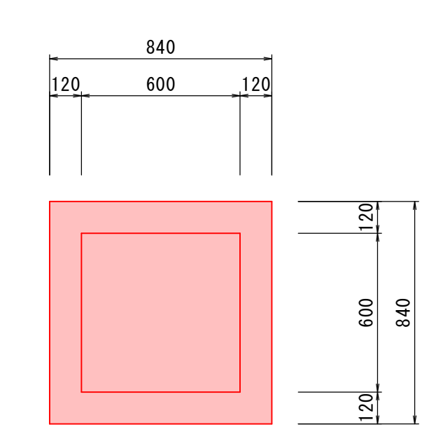
3号集水樹 プレキャスト集水樹 SM-B600-H700
