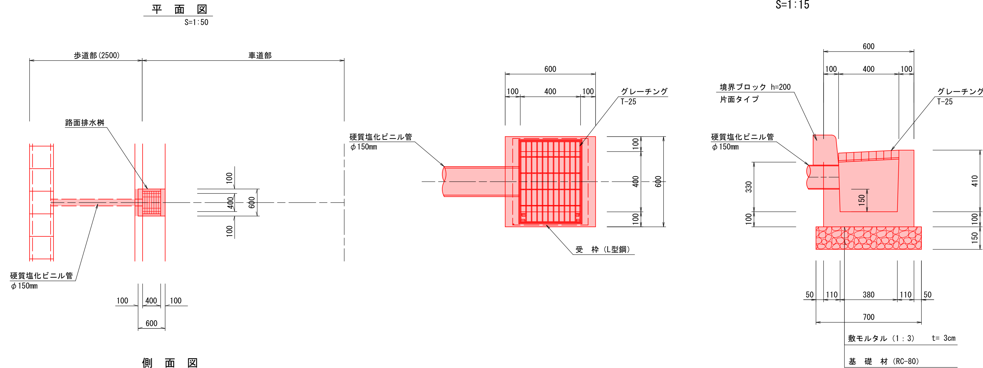
S=1:50 マウンドアップ標準タイプ
