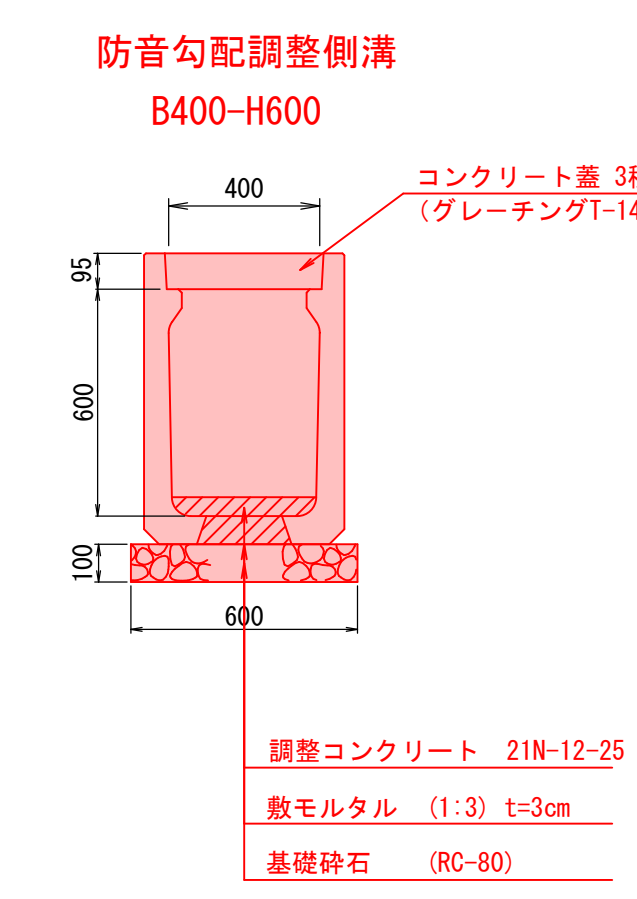
側溝構造図 S=1:20
