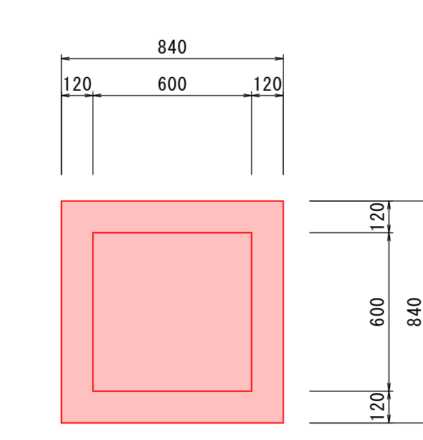
5号集水樹 プレキャスト集水樹 SM-B600-H700
