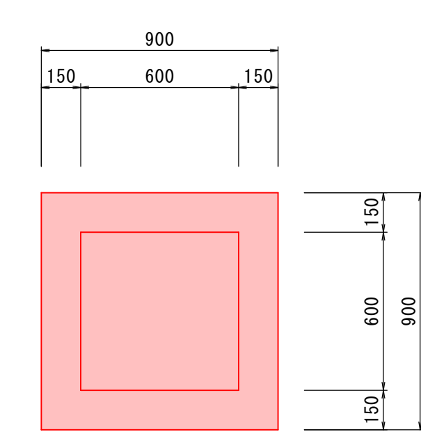
4号集水樹 場所打ち集水樹 SM-B600-H830
