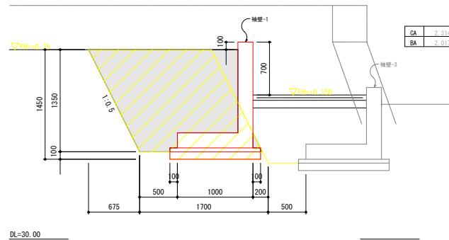
③-2断面図
