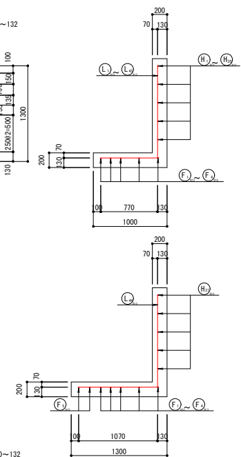
断面図
