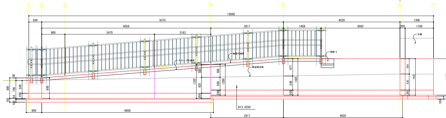
スロープ袖壁-3 展開図
