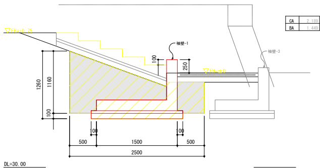
①断面図
