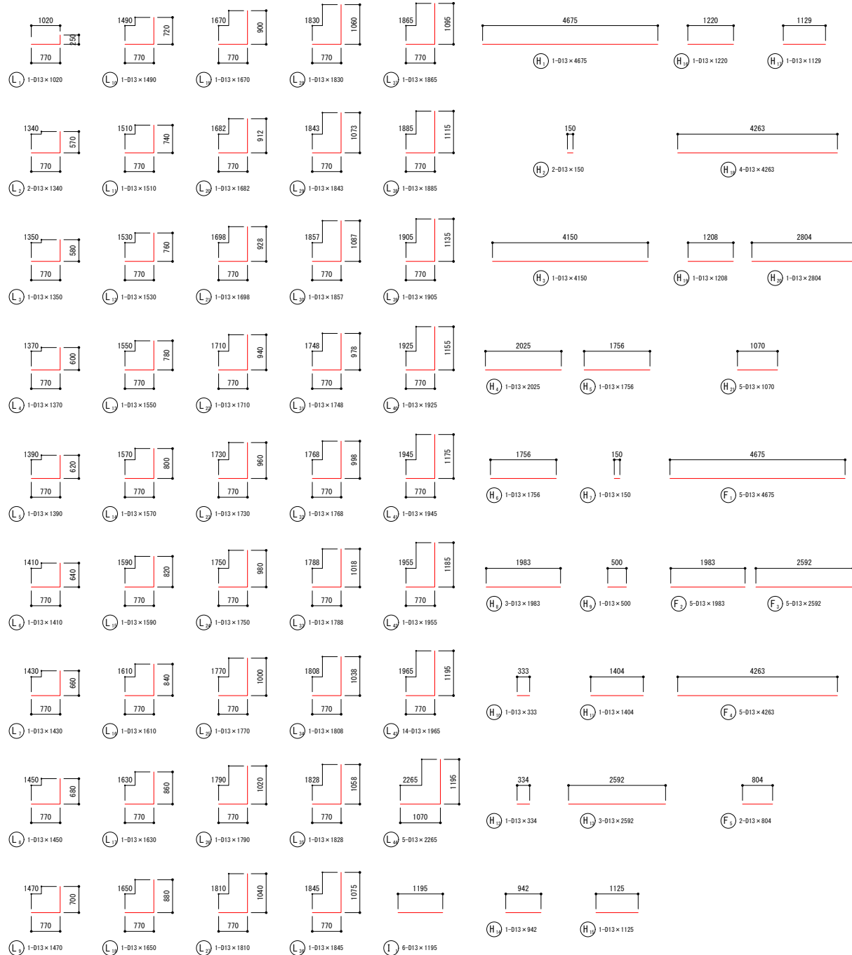
スロープ袖壁-3配筋図(2)
