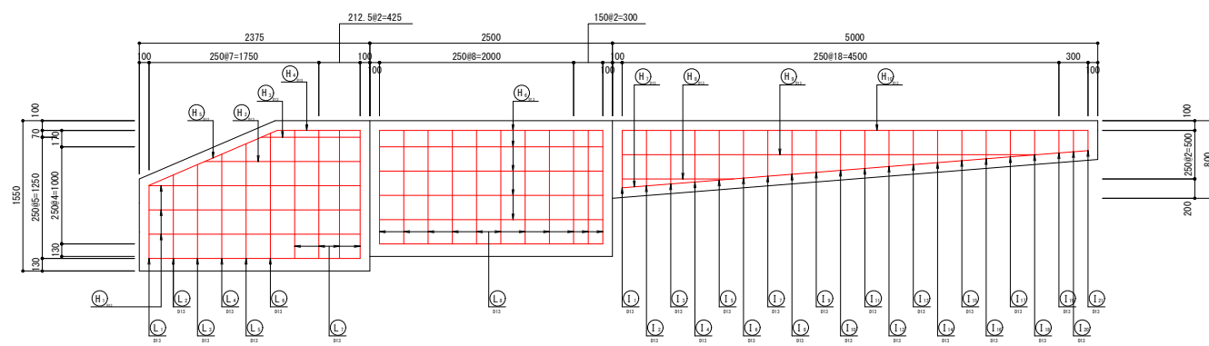
正面図
