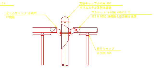
支柱取付部詳細図
