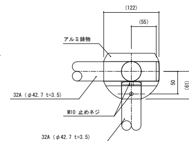
D部断面図 S=1:3 (A1) S=1:6 (A3)
