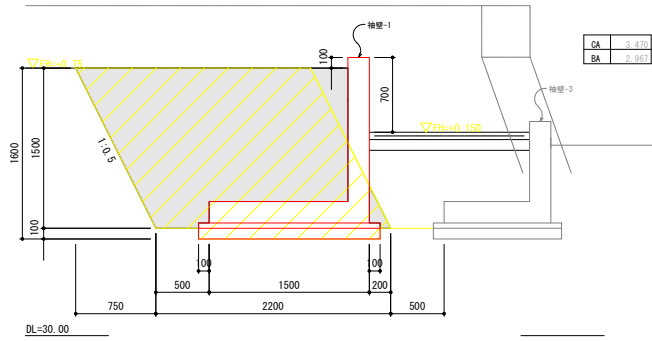
③-1断面図
