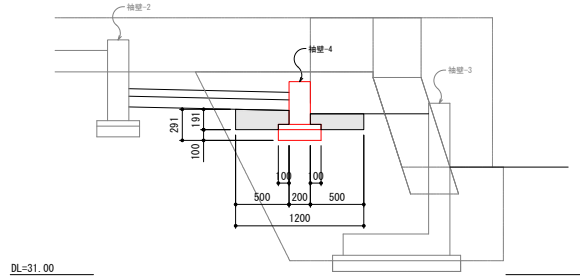
②断面図
