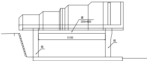
ステージ両端壁
