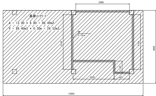
1 階 平 面 図
