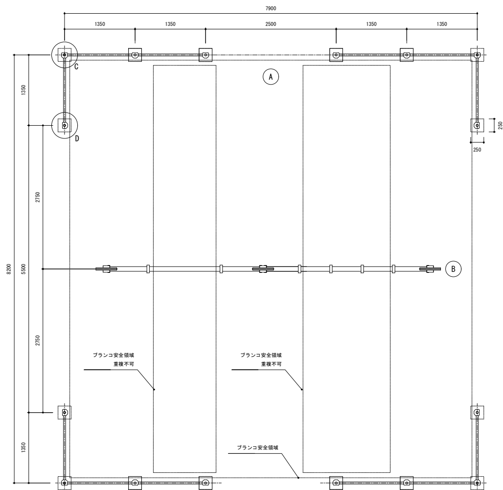
平面图 S=1:25
