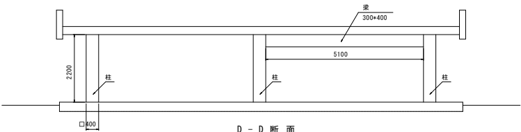
D - D 断面
