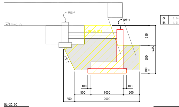
④-2断面図
