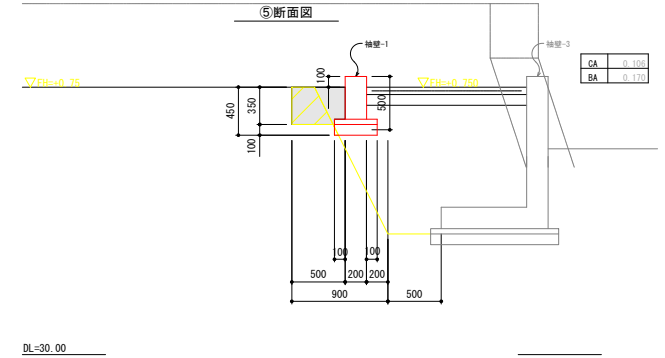
⑤断面図
