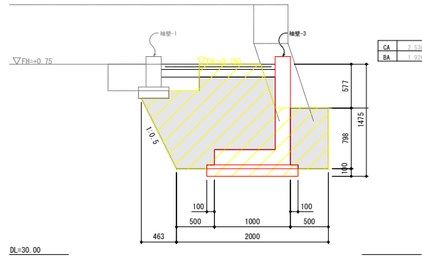
④-2断面図
