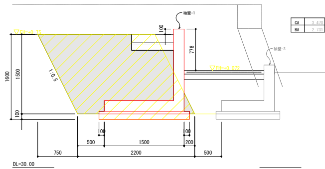
②断面図
