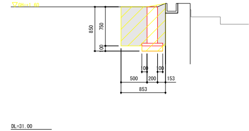
⑥断面図
