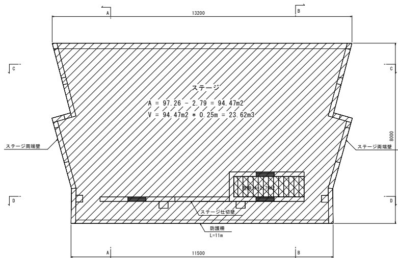
2 階 平 面 図
