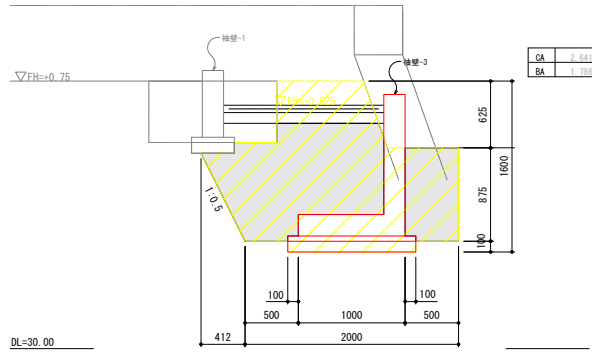
③断面図
