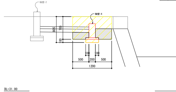
④-1断面図
