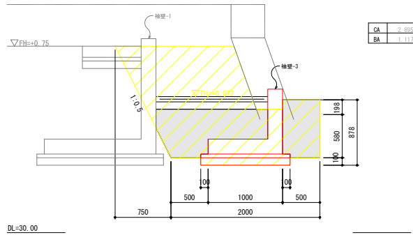
①・②断面図
