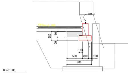
①断面図
