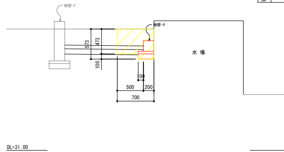
③-2断面図
