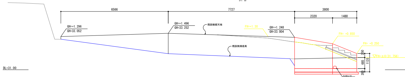
A-A' 展開図 S=1: 50
