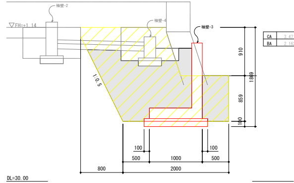
⑤断面図
