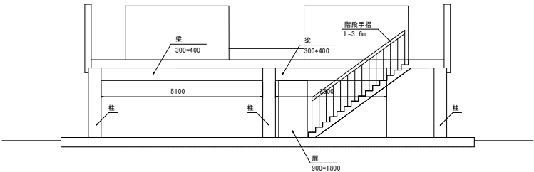
A - A 断面
