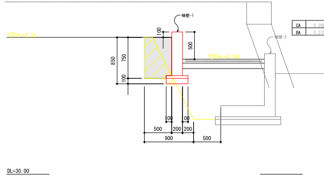
④-2断面図
