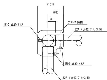
C部断面図 S=1:3
