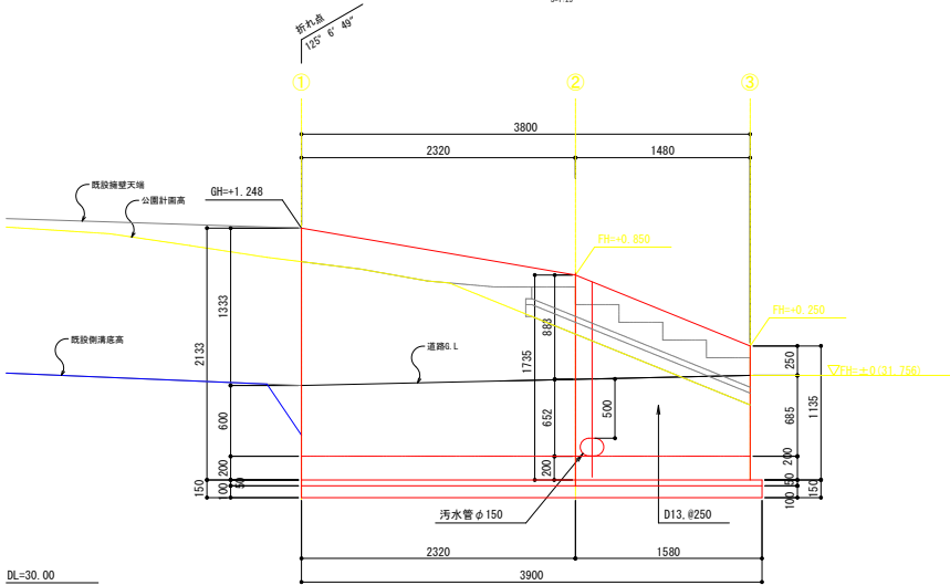
展開図
