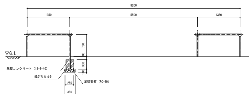
B部断面图 S=1:25
