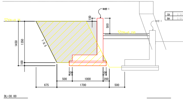
④-1断面図
