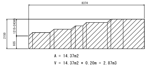
ステージ両端壁
