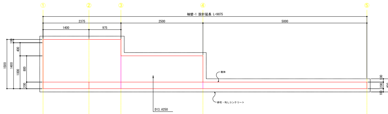
スロープ袖壁-1 平面図
