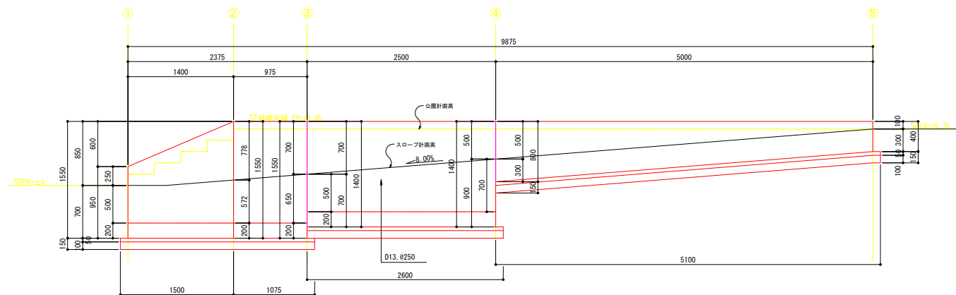
スロープ袖壁-1 展開図
