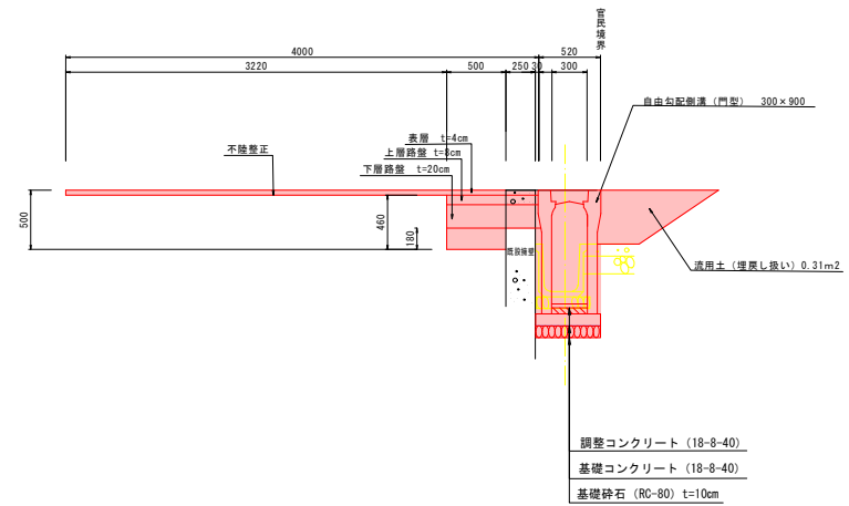
標準断面図（北側）
