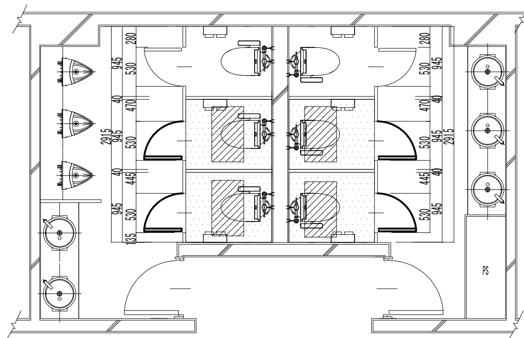
改修トイレ平面図
