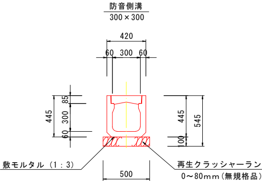
U型側溝一般図
