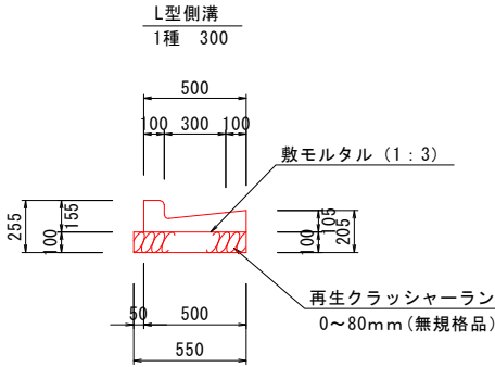
L型側溝一般図
