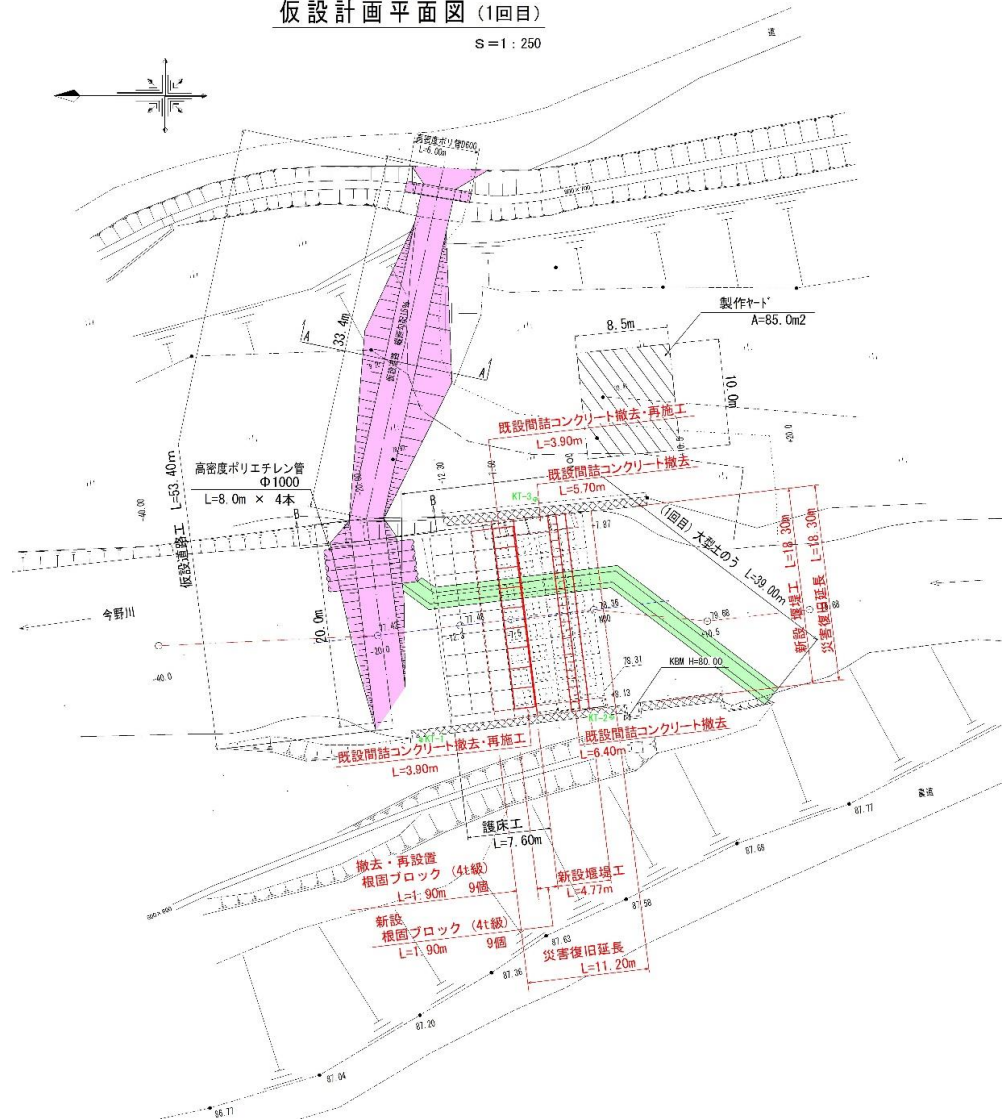
仮設計画平面図 (1回目)
