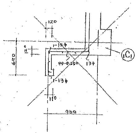
車庫入口袖機断面 S: 1/30
