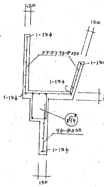
塔屋ホース掛場 S: 1/30
