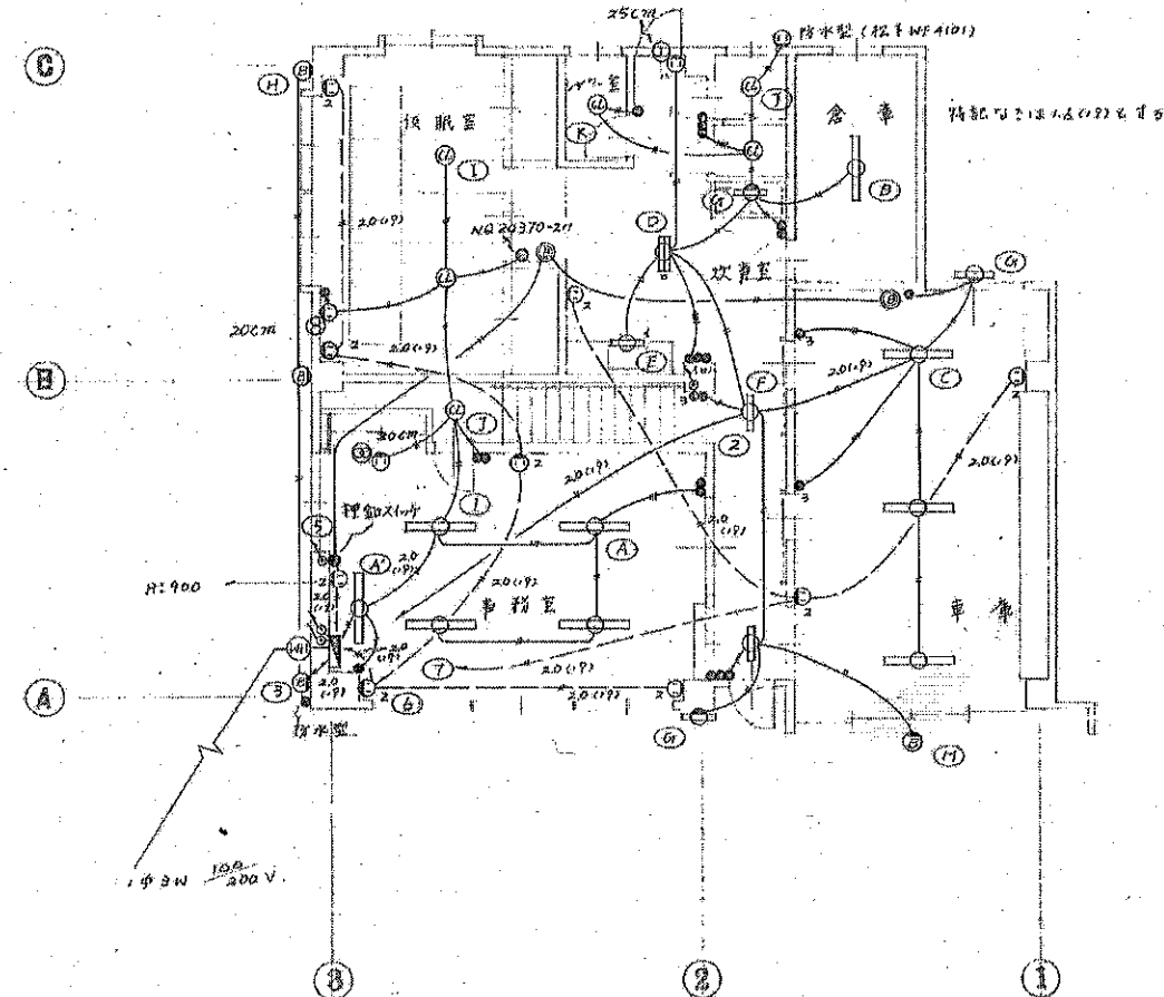
1階配線図
