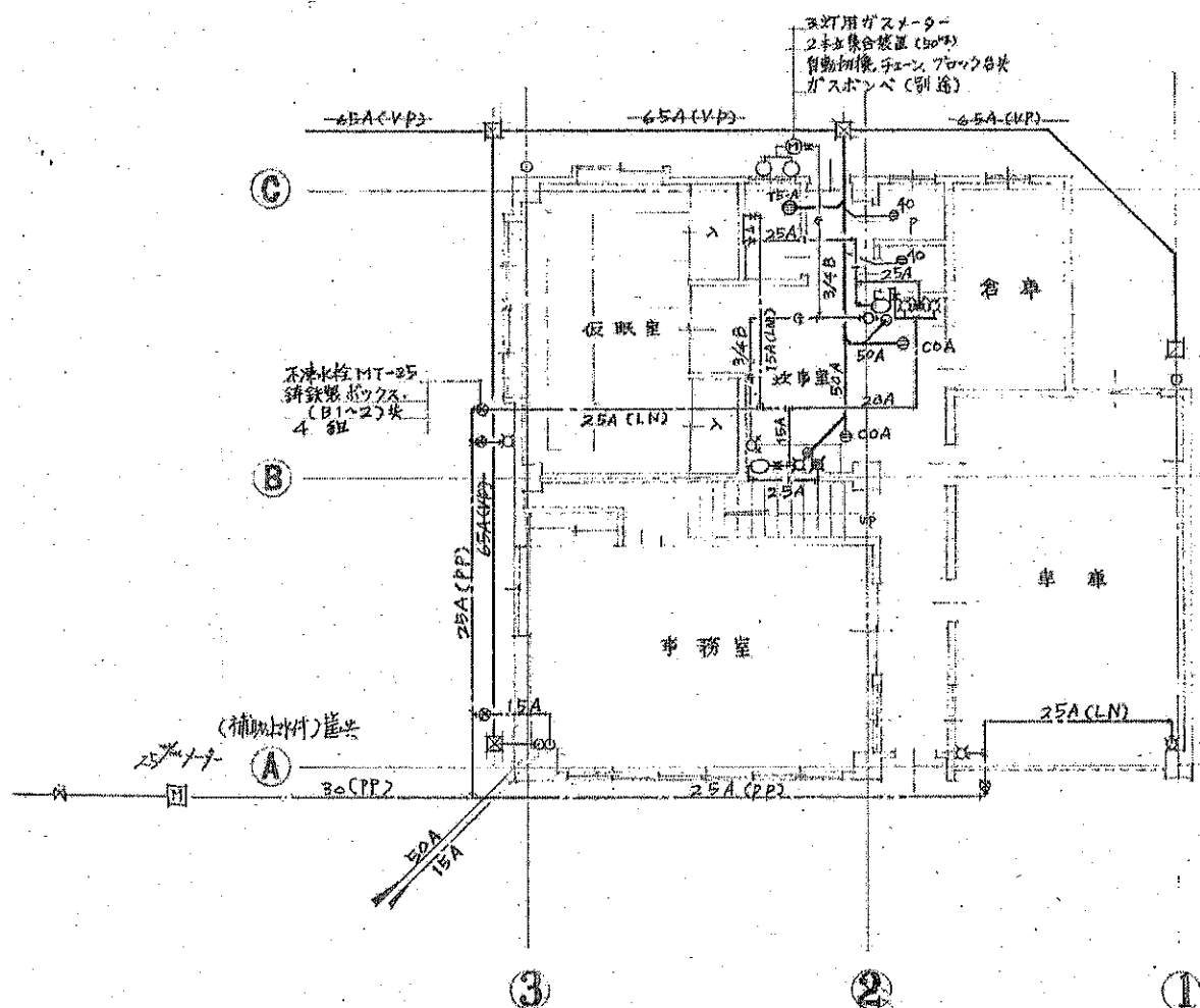
1階平面図
