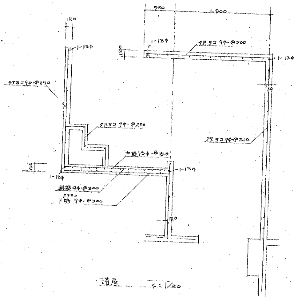
塔屋ホース掛場 S: 1/30
