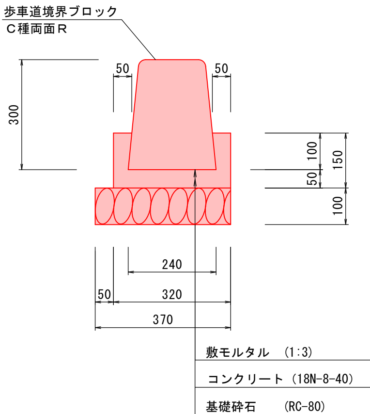
歩車道境界ブロック C種両面R B240-H300
