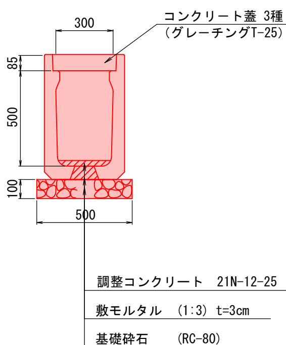
防音勾配調整側溝 B300-H500
