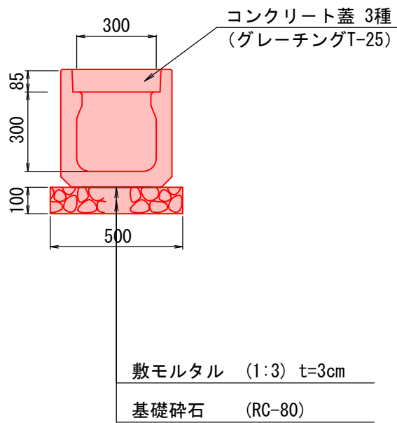
防音側溝 B300-H300
