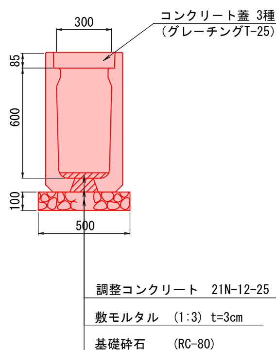
防音勾配調整側溝 B300-H600
