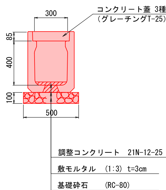
防音勾配調整側溝 B300-H400
