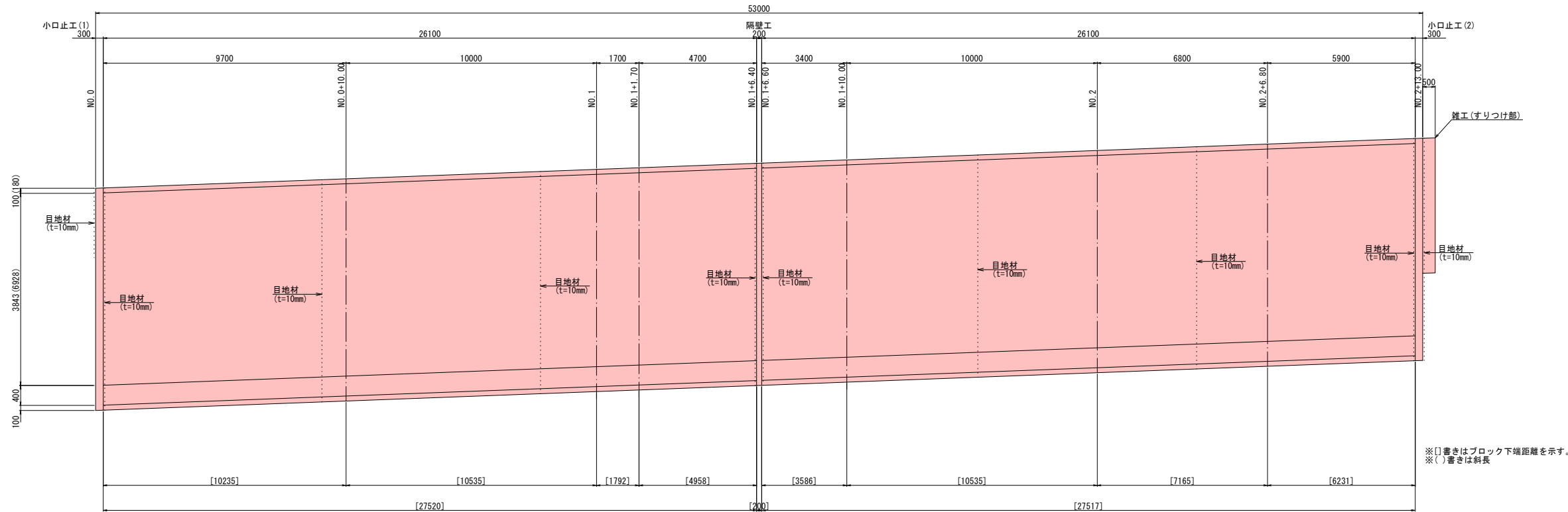
小口止工 S=1:50
