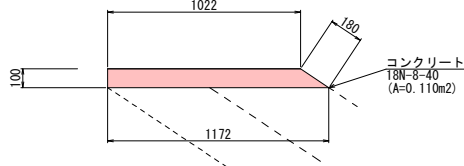
土台コンクリート詳細図 S=1:20
