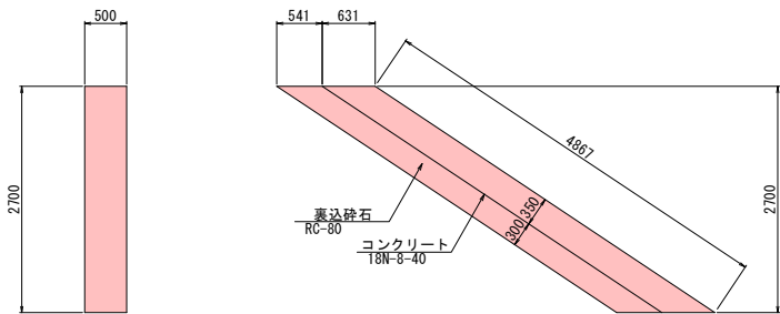
雑工(すりつけ部) S=1:50
