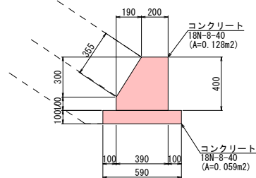
土台コンクリート詳細図 S=1:20
