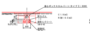
断面図 S=1:50
