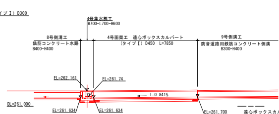
側面図 S=1:100
