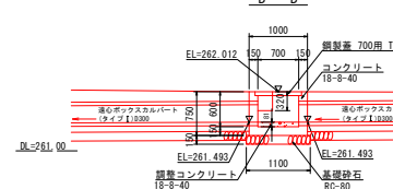
B-B
