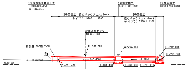
側面図 S=1:100
