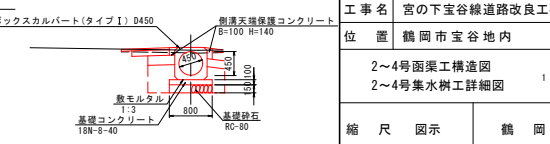
断面図 S=1:50
