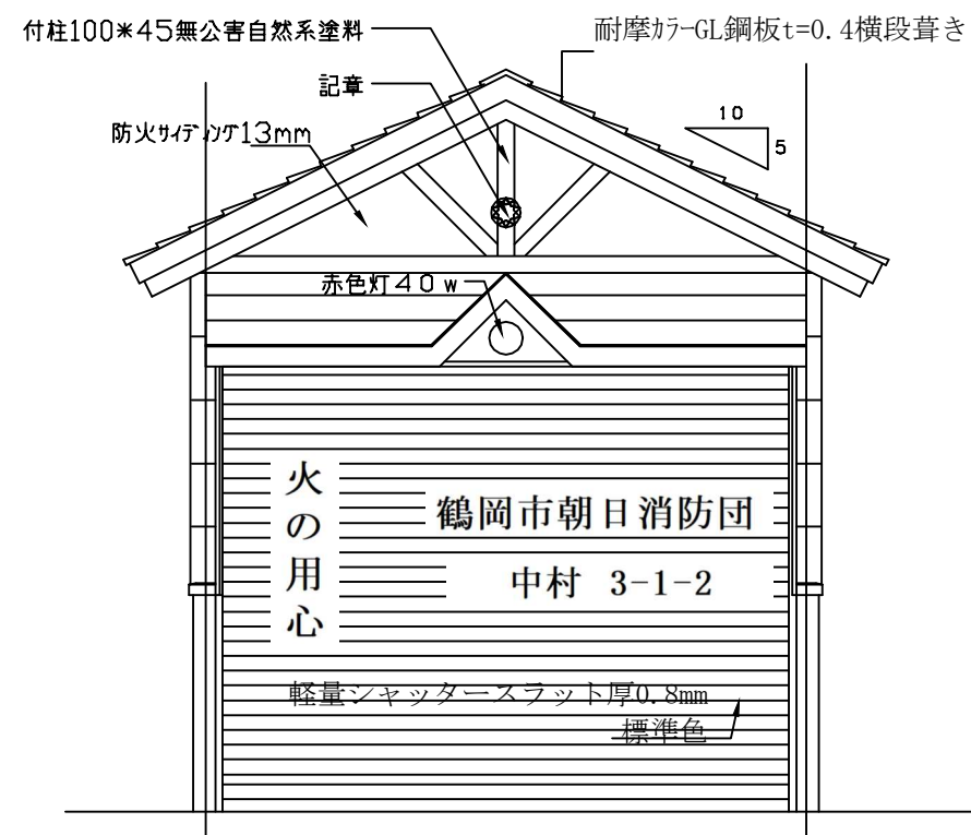
北側立面図
