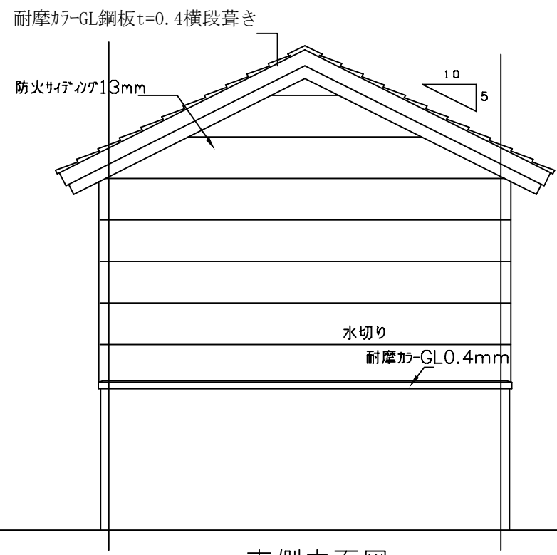
南側立面図
