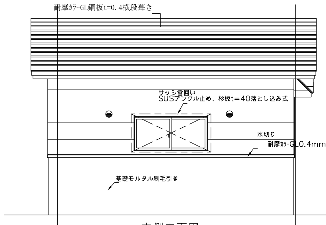
東側立面図
