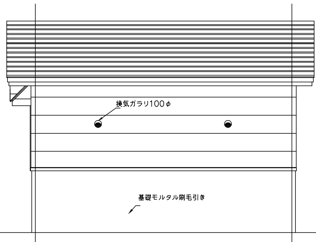
西側立面図
