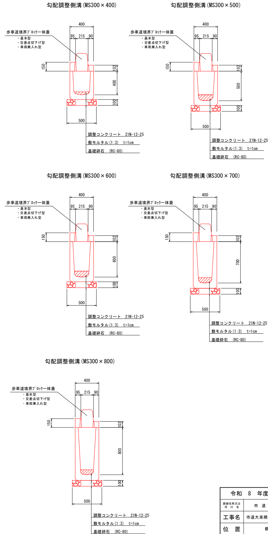
断面図 S=1:20
