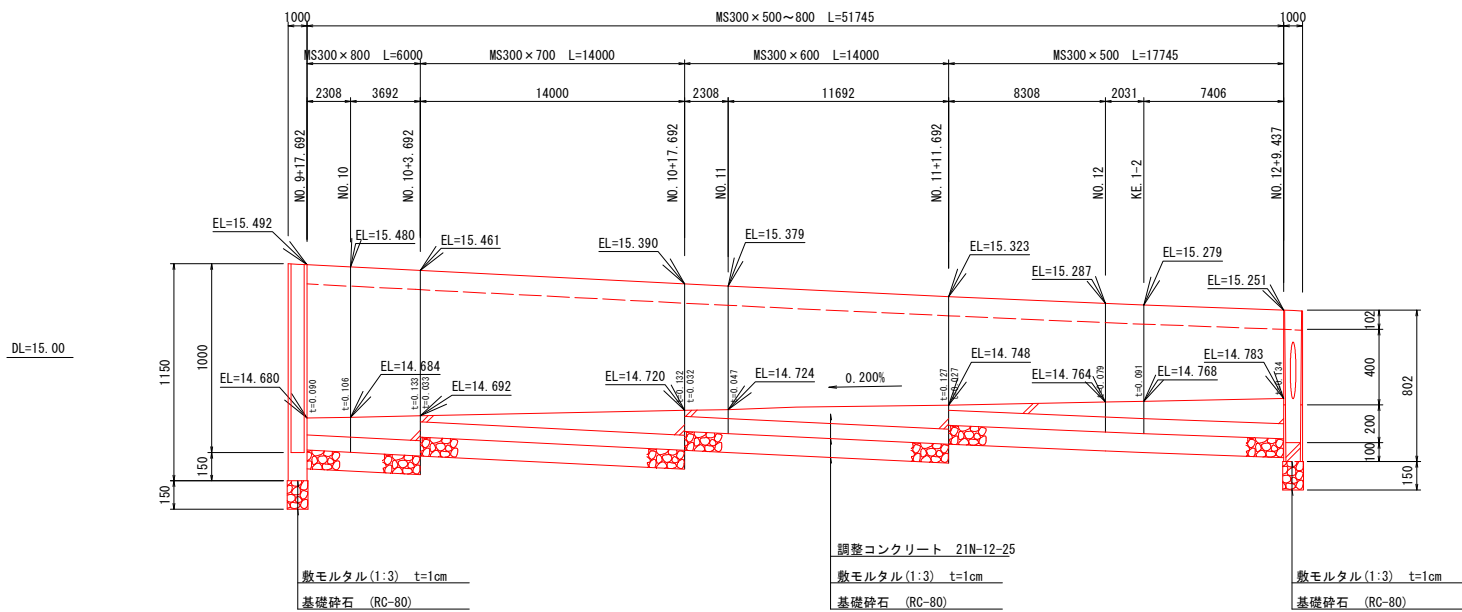
第4号勾配調整側溝側面図 (車線左側 NO. 9+17.692~NO. 12+9.437)
