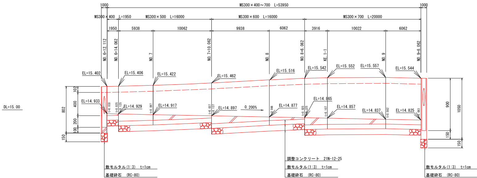
第2号勾配調整側溝側面図 (車線左側 NO. 6+12.112~NO. 9+6.062)
