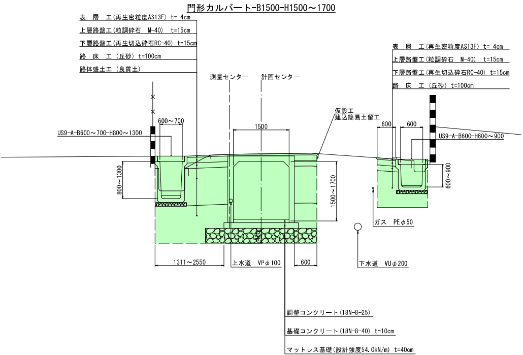
NO. 14+12. 89～NO. 28+11. 40 門形カルバート-B1500-H1500～1700
