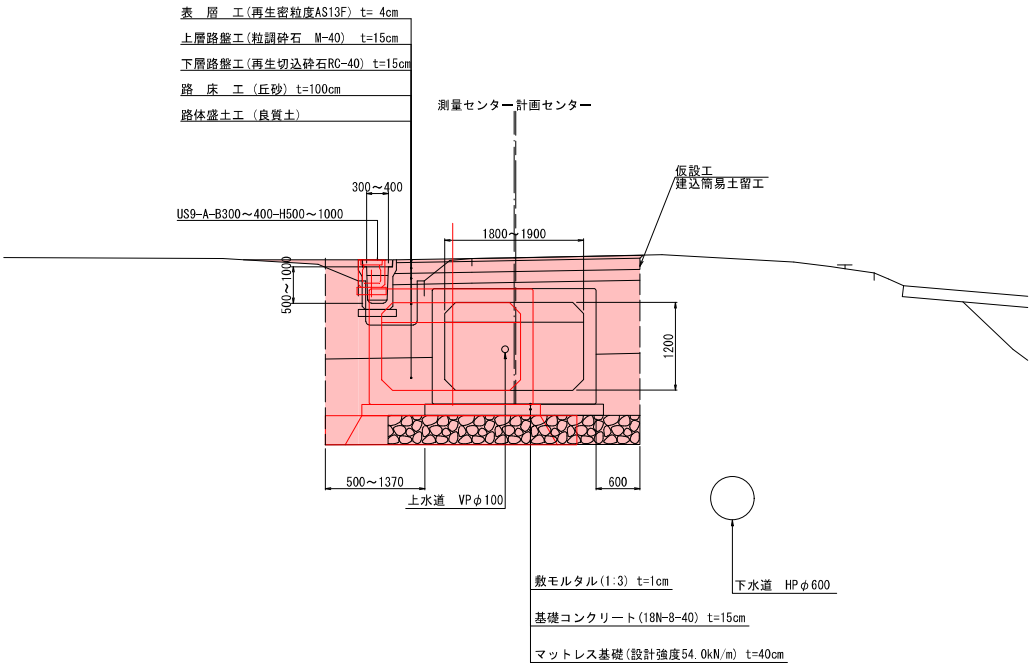
IP. 1～NO. 14+12. 89 RCB-B1800～1900-H1200
