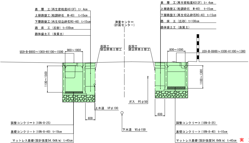
NO. 28+11. 40～NO. 46+1. 30 US9-B-B800～1000-H1100～1500
