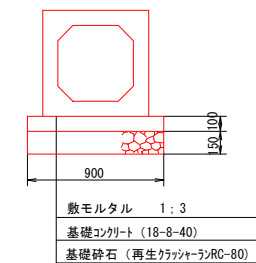
函渠工断面図 S=1:25
