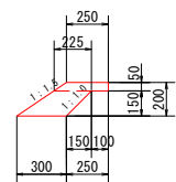
保護路肩工 S=1:25
