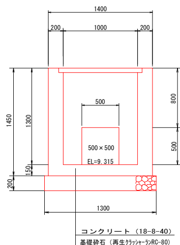
B-B断面
