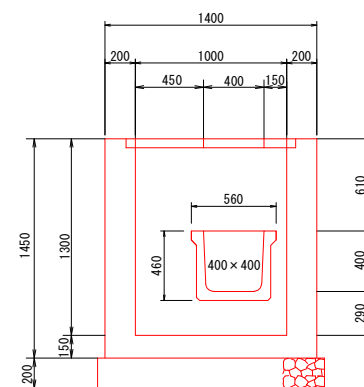
C-C断面
