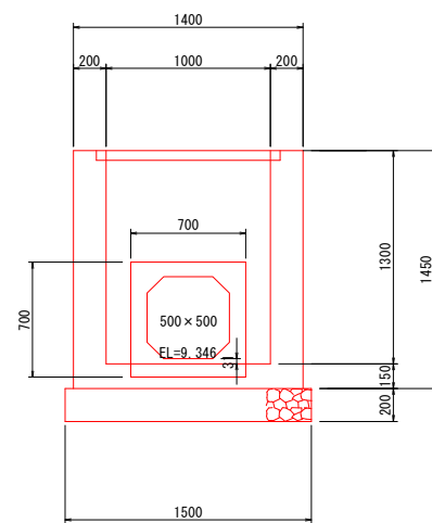
A-A断面
