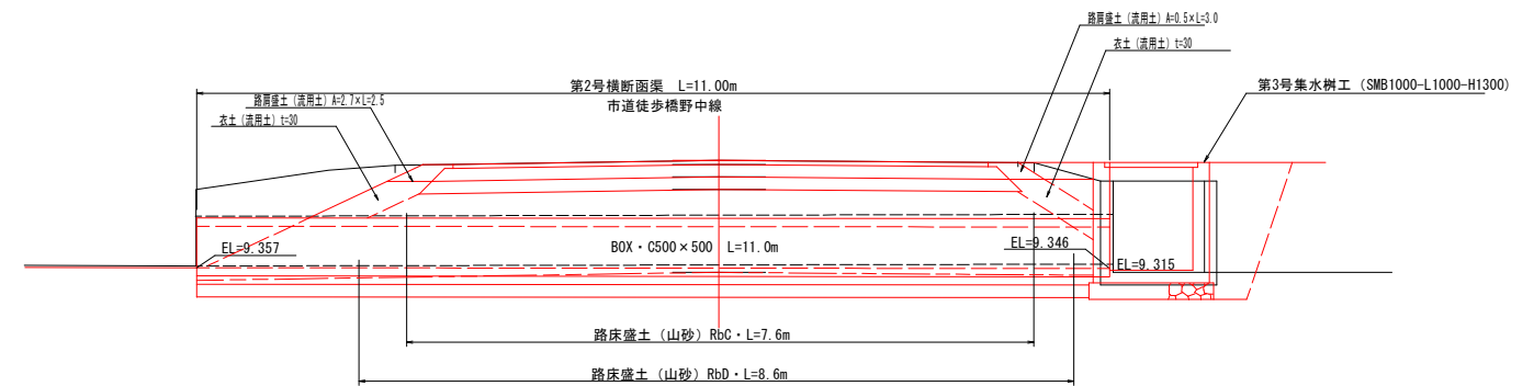
側面図 S=1:50
