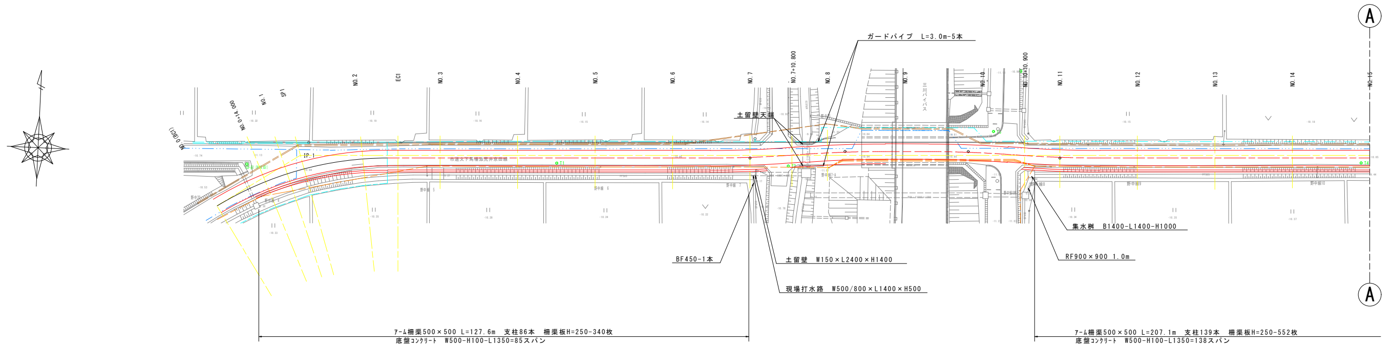
取壊し・撤去平面図 (参考図) S=1:500
