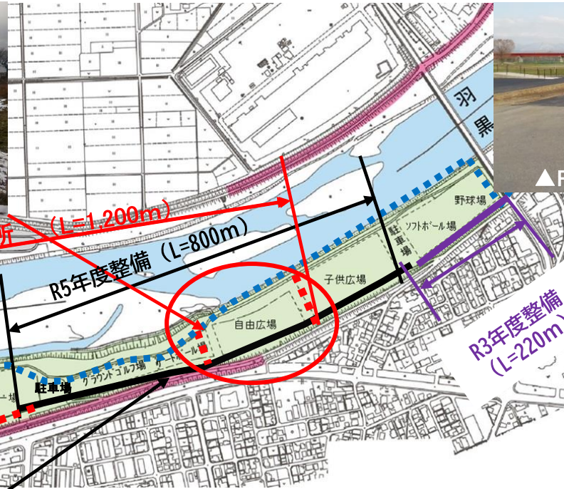
▲園路整備平面図
