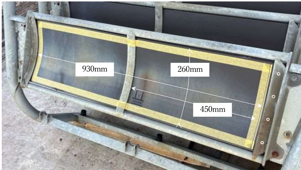
湯殿山スキー場第1ロマンスリフト搬器背面仕様図
