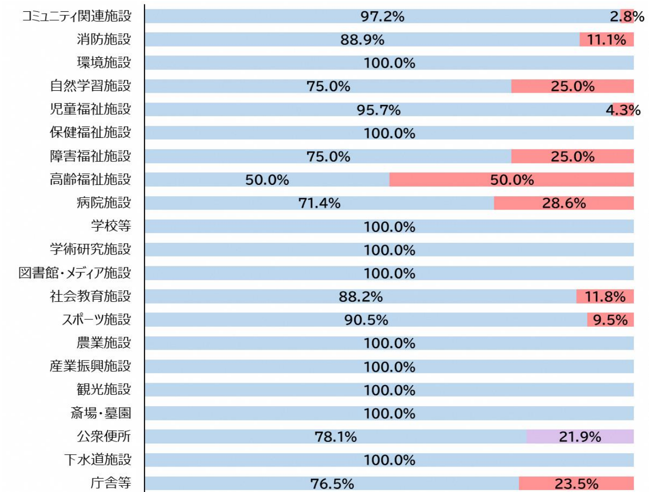
図5 建物系施設の施設類型別耐震化状況
