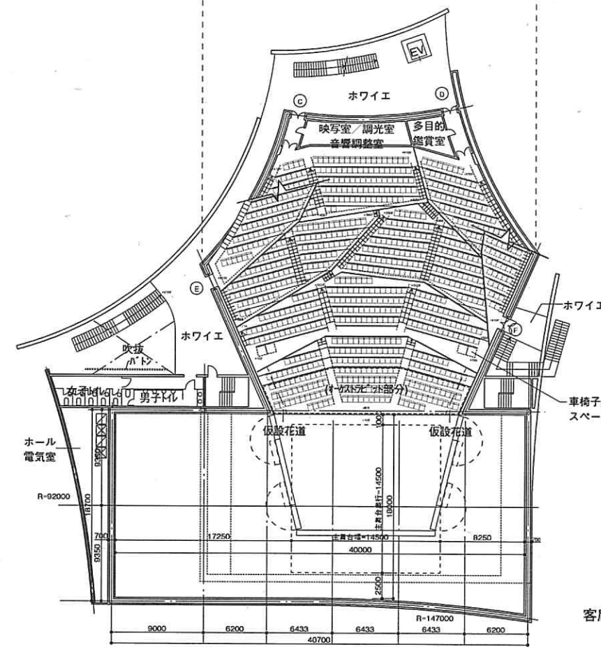
ホール部分平面図 1/500
