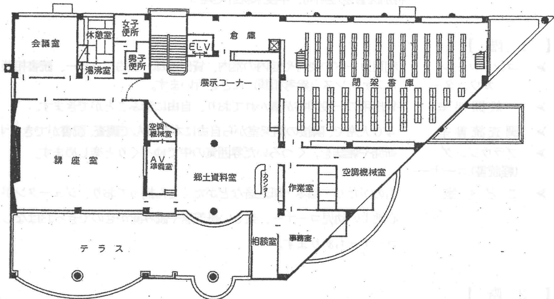
2階平面図
